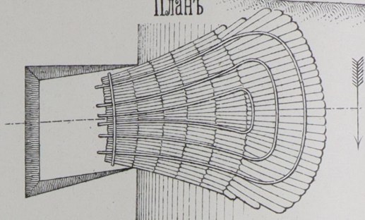
Планъ
