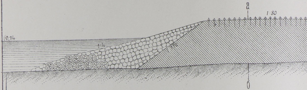
Черт. 1. Продольный разръзъ.
