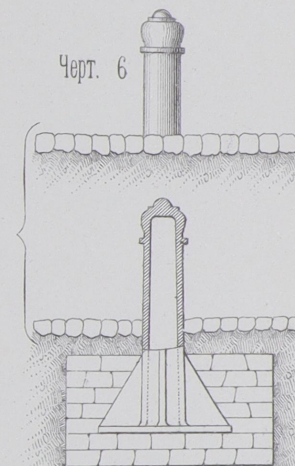
Разрѣзъ.
