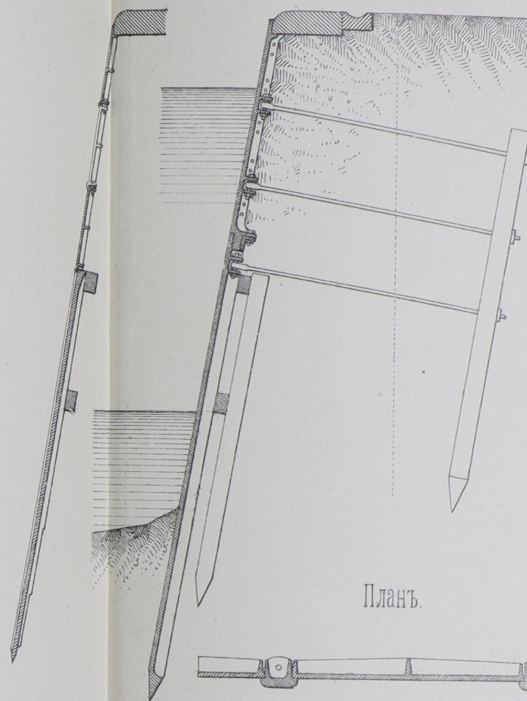
Разрѣзъ по А-В.
