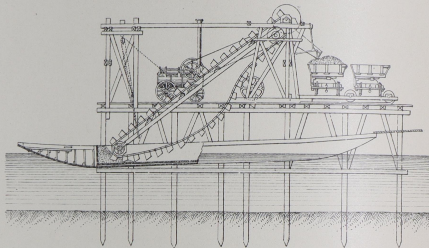
Планъ.
