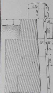
Разрѣзъ по А-В.
