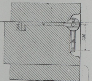
Планъ по шву.
