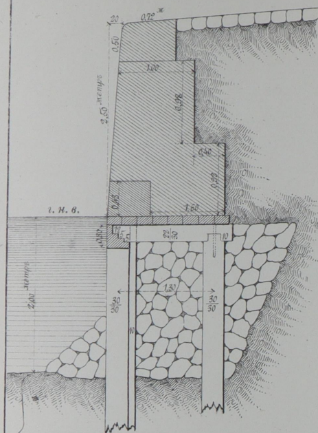
Черт. 8. Разрѣзъ по C-D.
