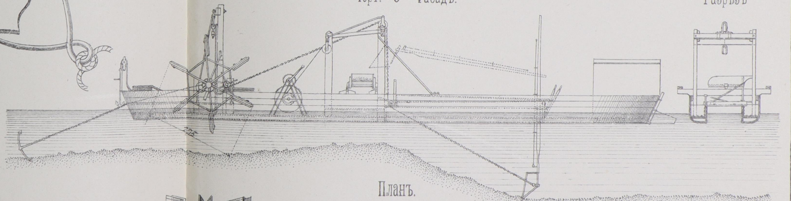
Черт. 6 Фасадъ.
