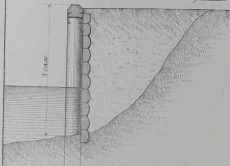
Разрѣзъ.
