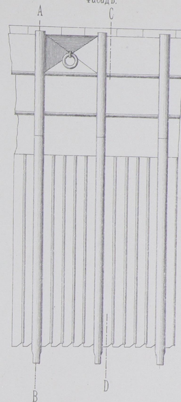
Фасадъ.
