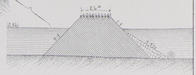
Разръзъ по а-б.
