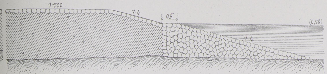
Черт. 5. Поперечный разръзъ.
