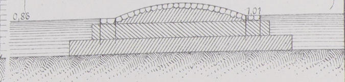
Разръзъ по а-б.
