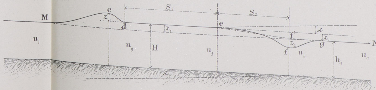
Черт. 8б. Продольная профиль по MN.
