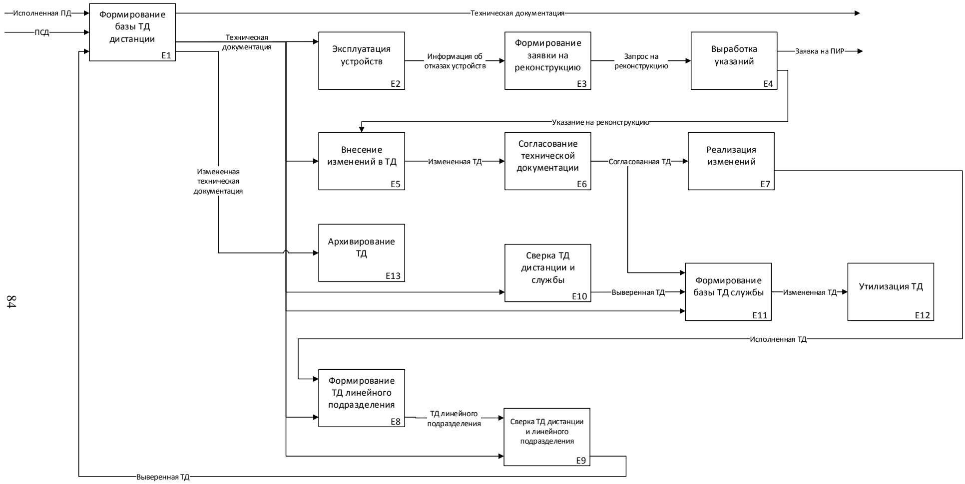
Рисунок 6 – Процесс эксплуатации объекта железнодорожной инфраструктуры
