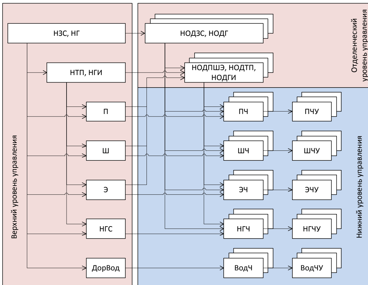
Рисунок 1 – Структура управления подразделениями, эксплуатирующими инфраструктуру
