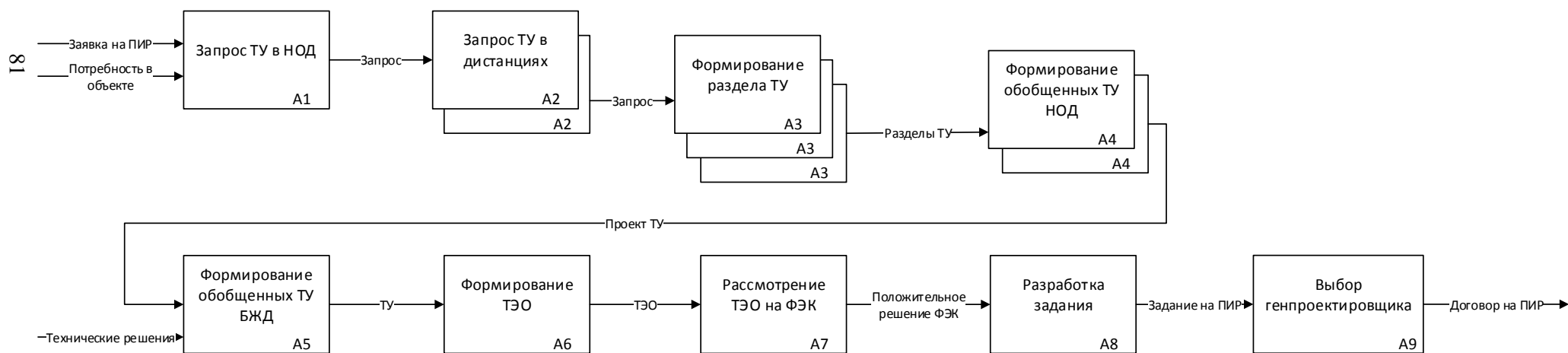
Рисунок 3 – Процесс заключения договора на проектно-изыскательские работы объекта железнодорожной инфраструктуры
