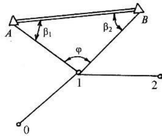
Рисунок 6.11 – Способ прямой угловой засечки
