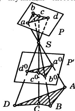
Рисунок 4.1 – Одиночный снимок и план объекта
