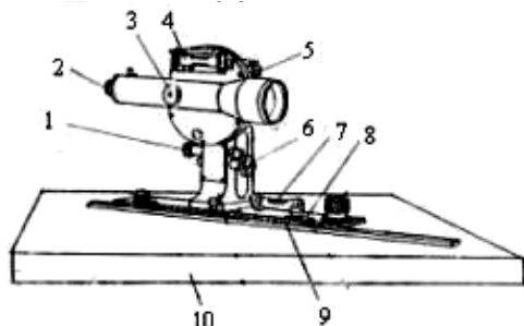
Рисунок 2.3 – Кипрегель КА-2
