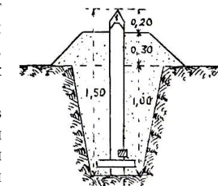
Рисунок 6.2 – Закрепление вершин углов поворота
