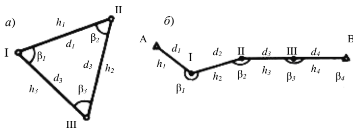
Рисунок 1.5 – Теодолитно-тахеометрические ходы: a – замкнутый; б – разомкнутый .
