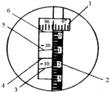
Рисунок 2.4 – Поле зрения кипрегеля КА-2: 1 – шкала вертикального круга; 2 – рейка; 3, 5 – номограммы превышений; 4 – номограмма горизонтальных проложений; 6 – основная кривая
