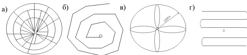
Рисунок 5.8 – Схемы съёмки пикетов при электронно-блочной тахеометрии: а – по радиусу; б – по спирали; в – лучевой; г – зигзагом
