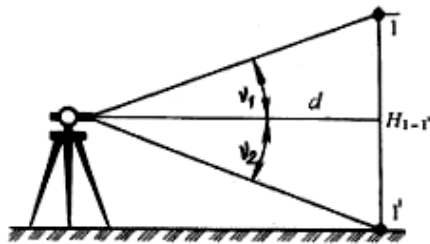
Рисунок 11.7 – Определение высоты
