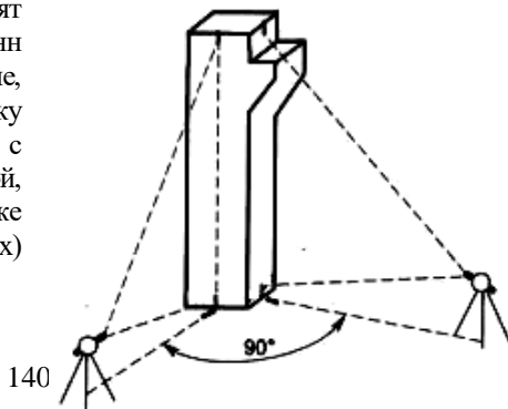
Рисунок 8.11 – Установка колонны
