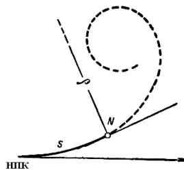
Рисунок 6.7 – Клотоида
