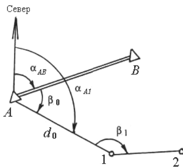
Рисунок 6.10 – Привязка трассы
