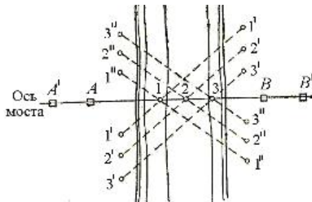
Рисунок 10.15 – Схема закрепления положения опор
