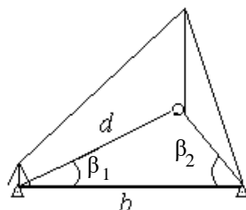
Рисунок 5.4 – Схема определения горизонтального проложения ковенным способом
