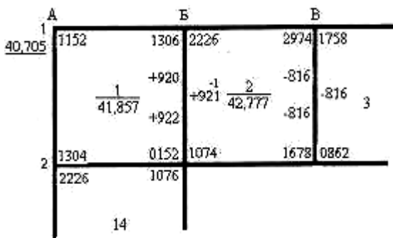
Рисунок 3.2 – Фрагмент журнала нивелирования поверхности по квадратам
