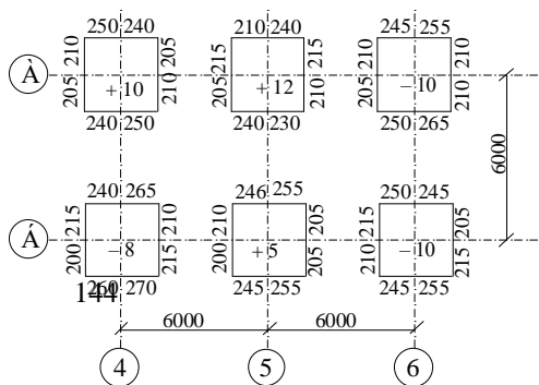
Рисунок 8.14 – Исполнительная съемка
