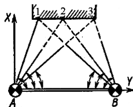
Рисунок 8.24 – Способ направлений
