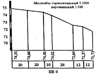
Рисунок 6.21 – Поперечный профиль
