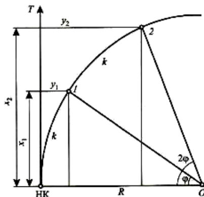
Рисунок 10.2 – Способ прямоугольных координат
