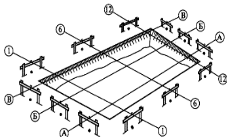
Рисунок 8.4 – Створная обноска
