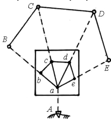
Рисунок 2.11 – Съемка ситуации
