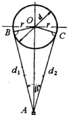
Рисунок 11.8 – Определение радиуса сечения
