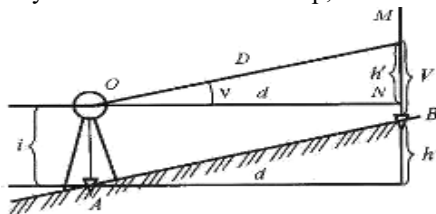
Рисунок 1.2 – Тригонометрическое нивелирование
