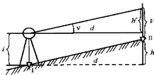
Рисунок 2.9 – Тригонометрическое нивелирование
