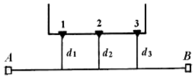
Рисунок 8.21 – Створный метод
