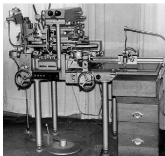
Рисунок 4.14 – Стереограф СД-3
