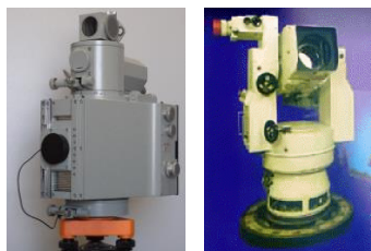
Рисунок 4.4 – Фототеодолиты
