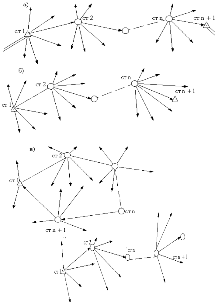
Рисунок 5.6 – Схемы последовательной электронно-блочной тахеометрии Другой особенностью электронно-блочной тахеометрии является то, что в ходовой линии (за ходовую линию принимается линия, проложенная
