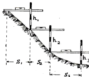
Рисунок 6.18 – Нивелирование крутого склона
