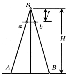
Рисунок 4.8 – Масштаб аэрофотоснимка
