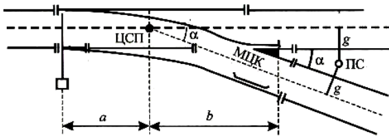
Рисунок 10.10 – Схема стрелочного перевода
