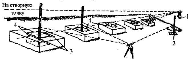
Рисунок 8.13 – Выверка положения фундамента
