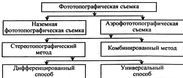
Рисунок 4.3 – Фотограмметрические методы, применяемые для создания планов и карт
