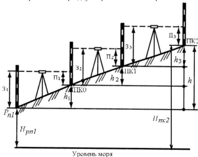
Рисунок 6.13 – Порядок нивелирования по трассе
