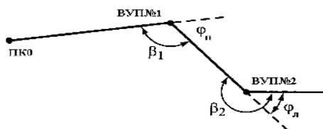
Рисунок 6.3 – Определение углов поворота по трассе
