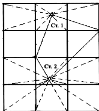
Рисунок 3.3 – Нивелирование через связующие точки
