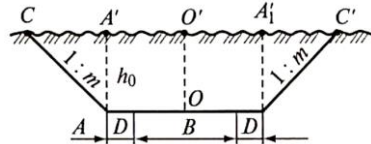
Рисунок 10.7 – Разбивка поперечника в выемке
