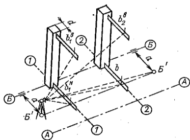
Рисунок 8.17 – Определение отклонения колонн
