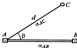
Рисунок 7.7 – Способ полярных координат
