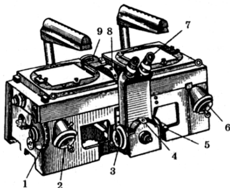
Рисунок 4.13 – Стереоскоп «Стеко 1818»
