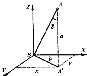
Рисунок 8.25 – Определение крена
