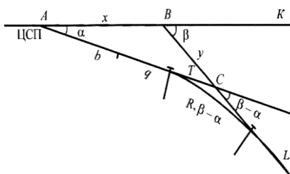
Рисунок 10.12 – Примыкание путей
