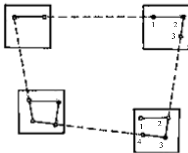
Рисунок 2.10 – Схема построения мензурного хода
