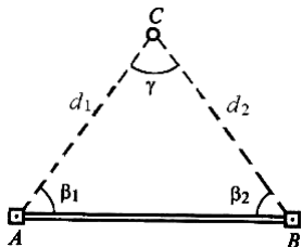
Рисунок 7.9 – Способ прямой угловой засечки
