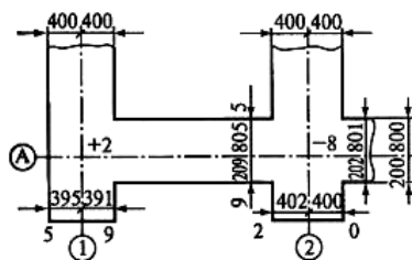
Рисунок 8.16 – Исполнительная съемка фундамента
