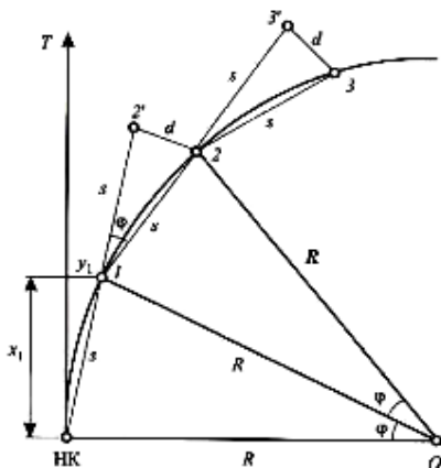
Рисунок 10.4 – Способ продолженных хорд
