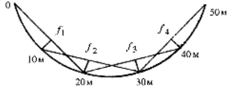
Рисунок 11.1 – Схема съемки по способу измерения стрел
