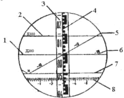
Рисунок 2.5 – Поле зрения кипрегеля КН: 1, 2 – номограммы горизонтальных проложений; 3 – рейка; 4 – вертикальный штрих; 5, 6 – номограммы превышений; 7 – основная кривая; 8 – шкала вертикального
