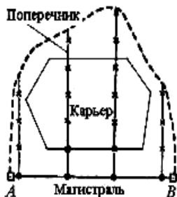
Рисунок 3.4 – Нивелирование по магистралям
