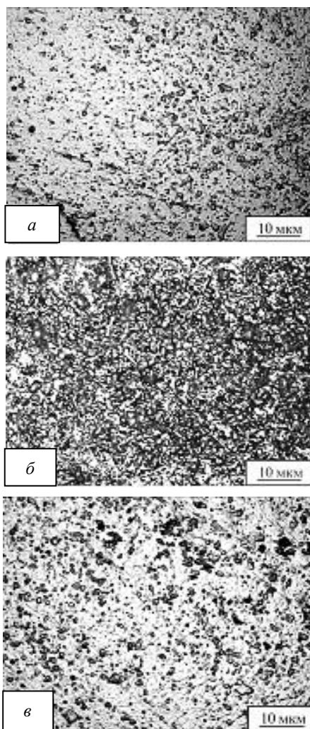
Рисунок 3 – Микроструктуры фольг из алюминиевых сплавов: а – Al-2,5% Cr-2,5% Zr, v = 30 м/с; б – Al-2,37% Cr-2,35% Zr, v = 40 м/с; в – Al-2,37% Cr-2,35% Zr, v = 50 м/с
