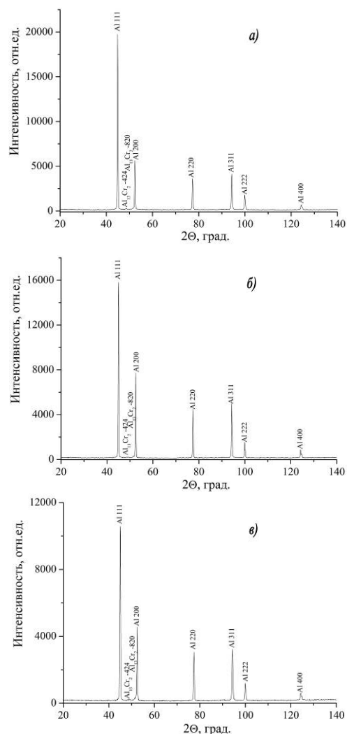
Рисунок 4 – Фрагменты рентгеновских дифрактограмм ( CoK_{\alpha} ) от поверхностных слоев алюминиевых сплавов: а – Al-2,5% Cr-2,5% Zr, v = 30 м/с; б – Al-2,37% Cr-2,35% Zr, v = 40 м/с; в – Al-2,37% Cr-2,35% Zr, v = 50 м/с
