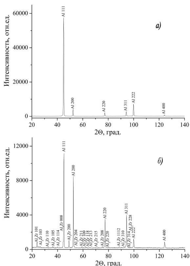
Рисунок 2 – Фрагменты рентгеновских дифрактограмм ( CoK\alpha ) от поверхностных слоев сплавов системы Al-Zr : а – Al-1,5\%Zr ; б – Al-5\%Zr , v = 30 м/с
