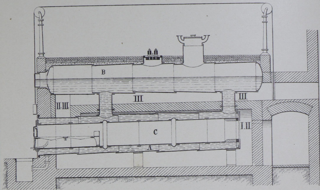
Черт. 24 а. Продольный разръзъ.
