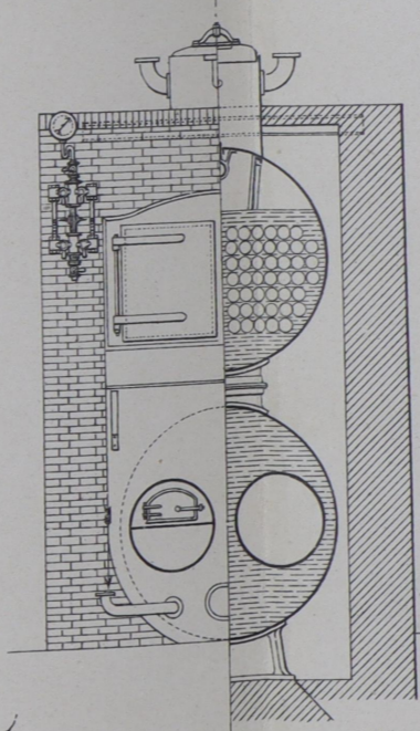
Черт. 26 б. Фасадъ и разръзъ по f e.
