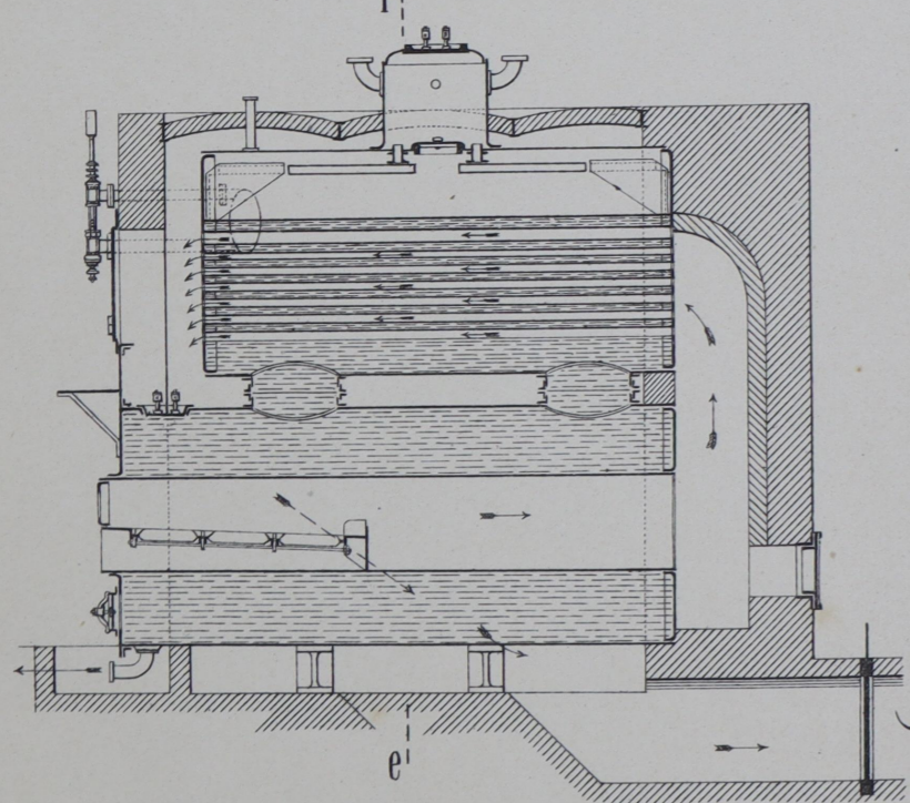
Черт. 26 а. Продольный разръзъ.
