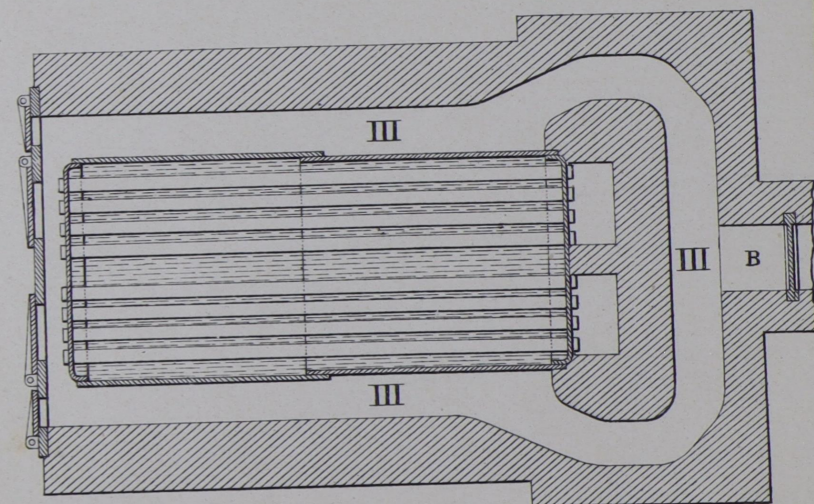
Черт. 25 в. Планъ.
