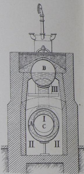
Черт. 24 б. Поперечный разръзъ.
