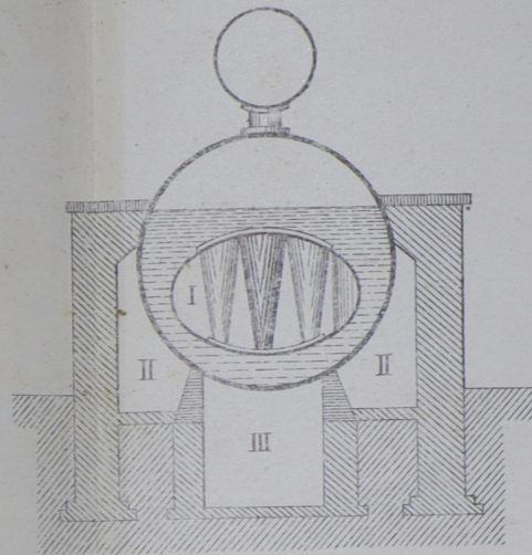
Черт. 16 а. Разръзъ по а с.
