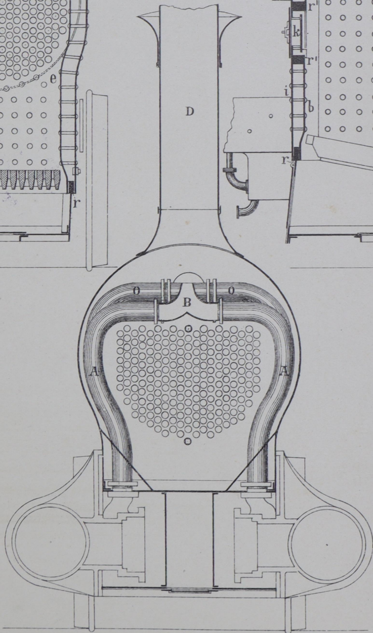
Черт. 31 в. Разрѣзь по γ δ.
