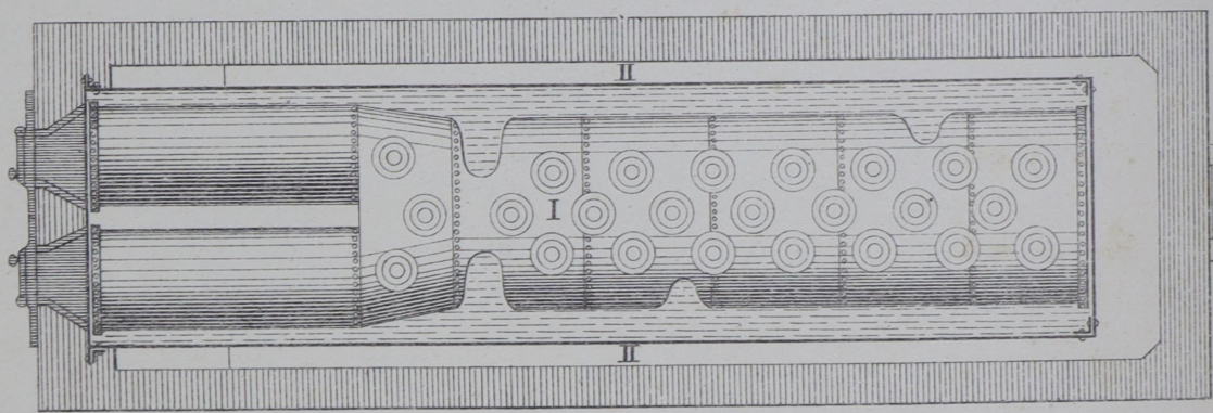
Черт. 22 в. Планъ.
