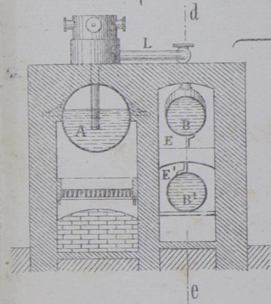
Черт. 16 а. Разръзъ по а с.
