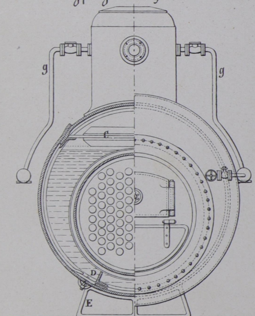
Черт. 28 б. Разрѣзь и фасадъ.
