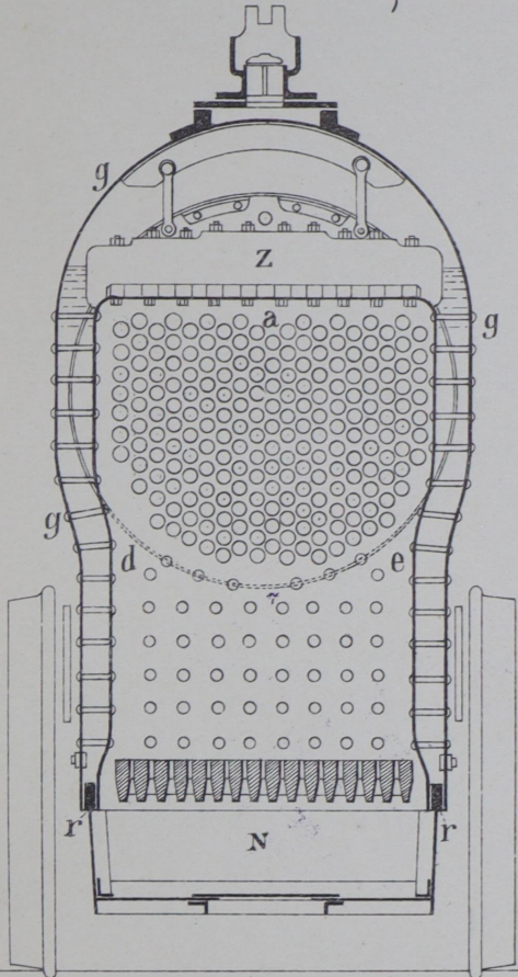
Черт. 31 б. Разрѣзь по а б.
