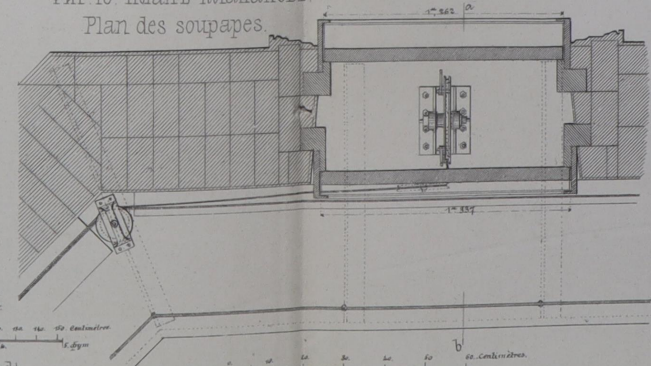
ОТОПЛЕНІЕ И ВЕНТИЛЯЦІЯ АНДРЕЕВСКАГО СОВОРА ВЪ С т ПЕТЕРБУРГѢ. CHAUFFAGE ET VENTILATION DE LA CATHÉDRALE S т ANDRÉ A S т PETERSBOURG.
