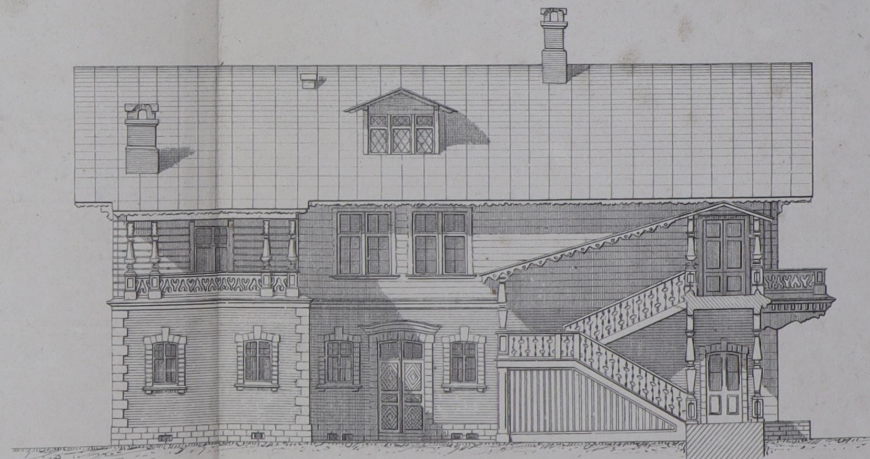
№2 БОКОВОЙ ФАСАДЪ И РАЗРѢЗЪ ПО АВ
