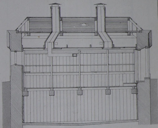
№4 ПРОДОЛЖИТЕЛЬНЫЙ РАЗРѢЗЪ ПО СД
