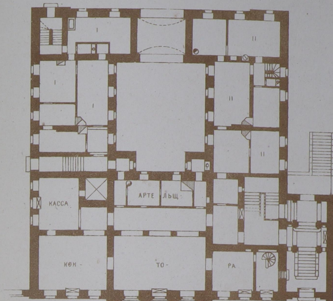
1 ЭТАЖЪ
