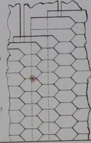
№ 11 Драневая кровля въ планѣ
