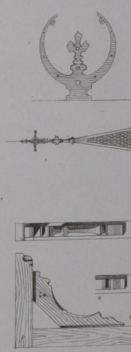
КОНСТРУКЦІЯ ГЛАВНАГО КАРНИЗА 1/4 НАТУРЫ
