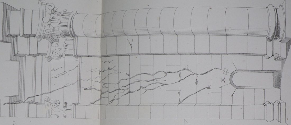
№ 2 Направление трещинъ въ контрфорсѣ X. Direction des crevasses et contrefort X
