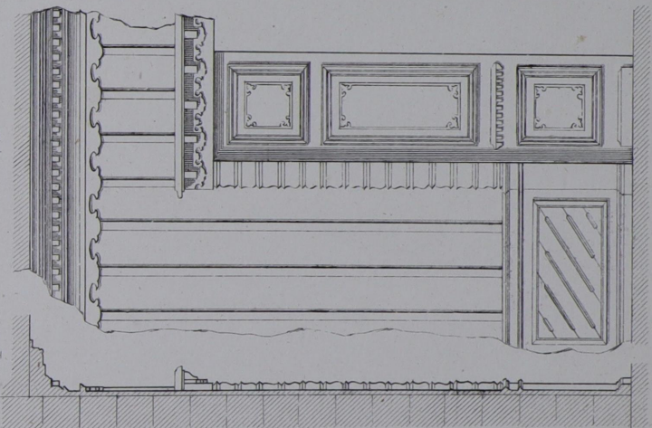
№4 Обшивка и дверь Гостиницы. б. Разрѣзъ
