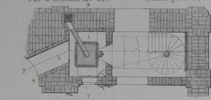
Фиг. 3. Разрѣзъ по r s. Coupe par r s.
