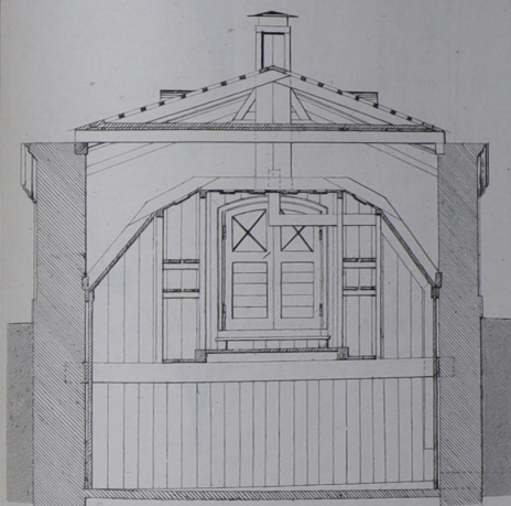
№3 ПОПЕРЕЧНЫЙ РАЗРѢЗЪ ПО АВ
