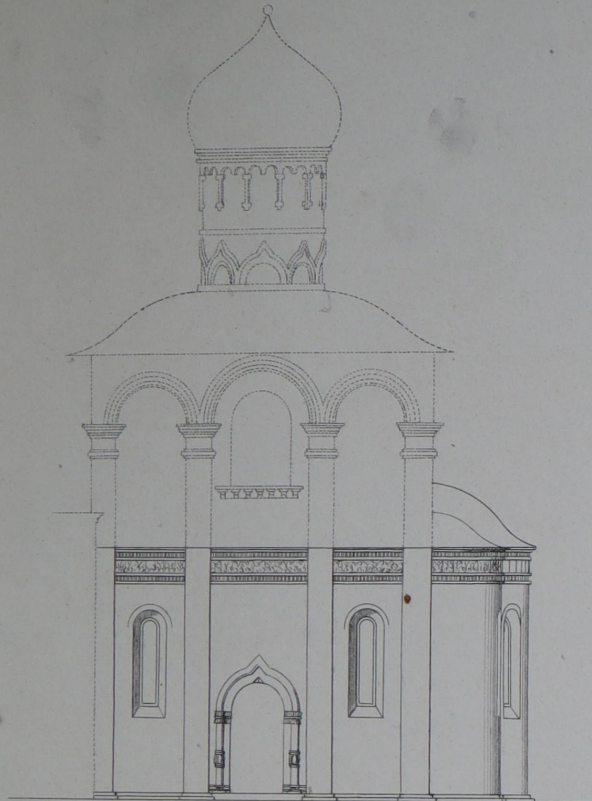
№ XII. Церковь Рождества Богородицы, въ старомъ Симоновѣ.
