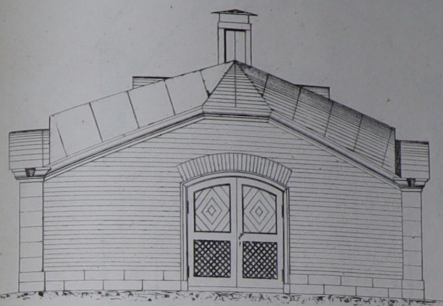
№1 ЛИЦЕВОЙ ФАСАДЪ
