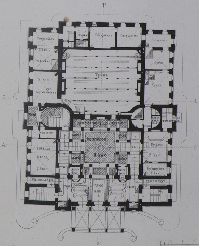
ПЛАНЪ НИЖНЯГО ЭТАЖА
