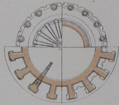
ПЛАНЪ ФОНАРЯ. PLAN DE LA LANTERNE
