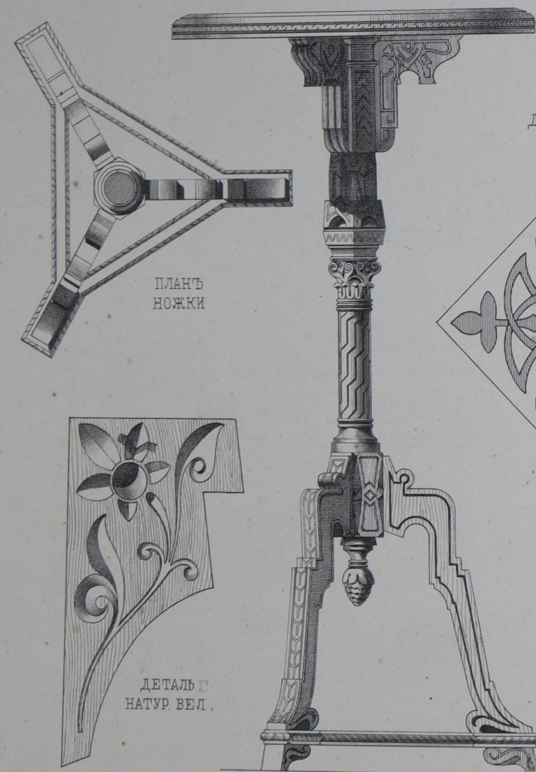
ГЕРИДОНЪ
