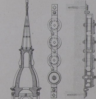
Фиг. 12. Проводы веревокъ для открыванія клапановъ. Conduits des cordes pour ouvrir les soupapes.
