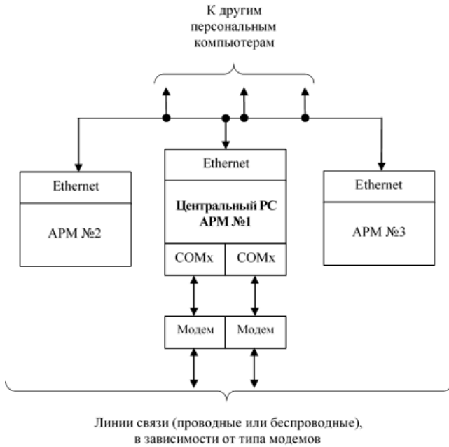
Рисунок 4.9 – Базовая структурная схема ПТК ЦПУ АСУДД
