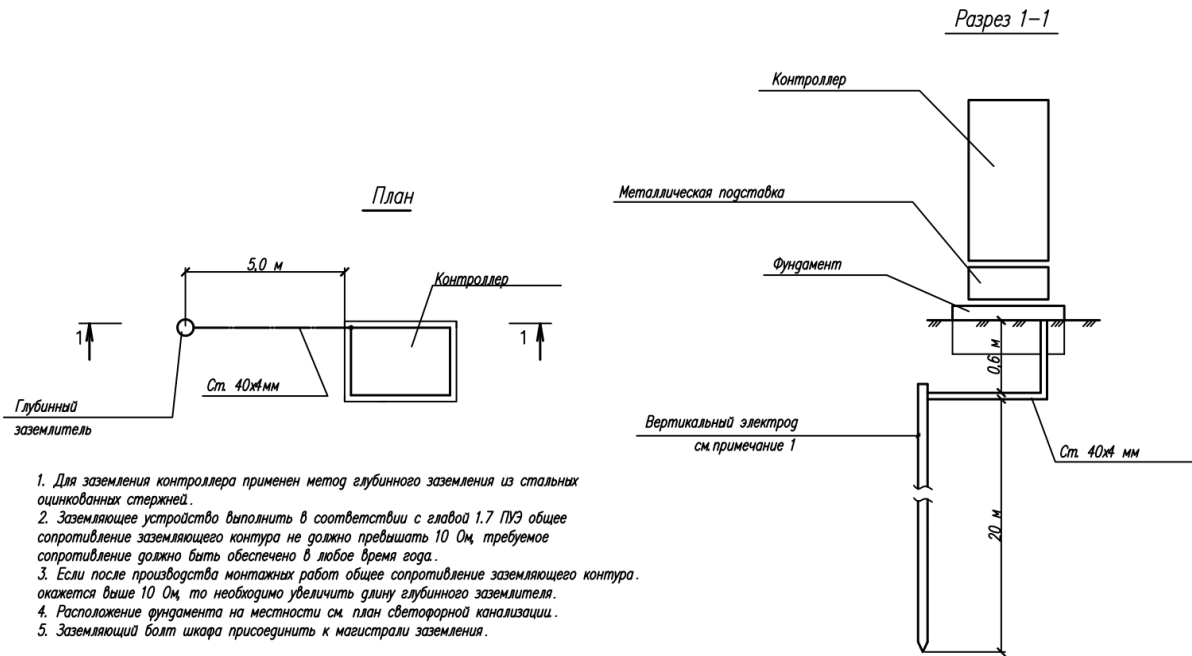
Рисунок 3.48 – Пример схемы устройства заземления ДК
