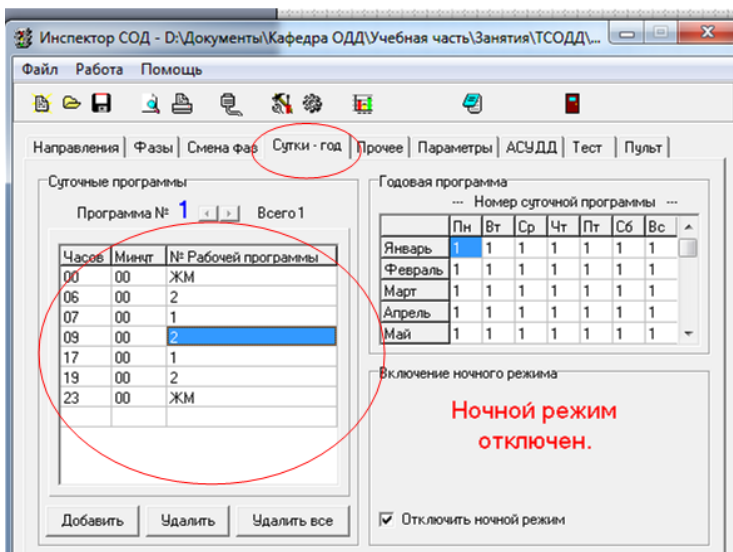
Рисунок 3.45 – Задание режима работы светофорного объекта по часам суток
