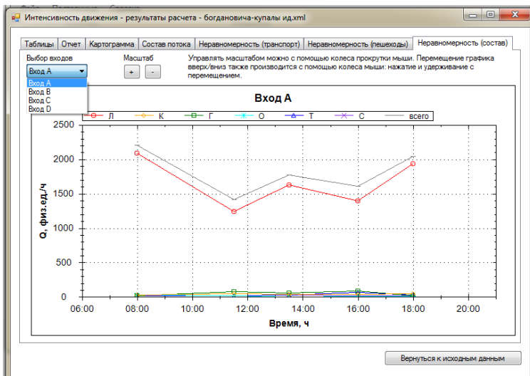
Рисунок 3.60 – Окно «Неравномерность (состав)» с графиками изменения состава транспортного потока на входе А по времени суток
