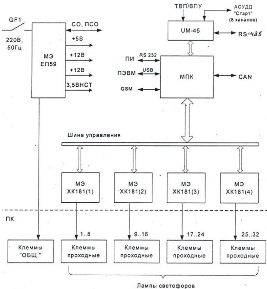
Рисунок 3.35 – Структурная схема БДКЛ-М в вариантах исполнения от БДКЛ-М-8с1 до БДКЛ-М-32с4
