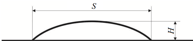
Рисунок 3.63 – Схема конструкции ИН 1 криволинейной формы
