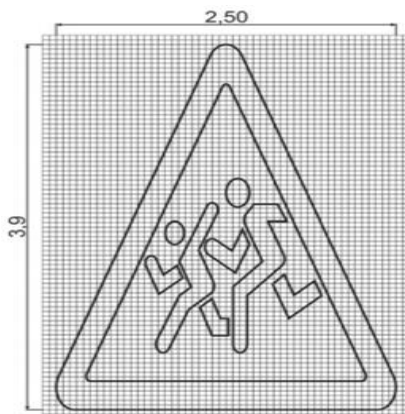
Рисунок В.8 – Горизонтальная разметка 1.24.2
