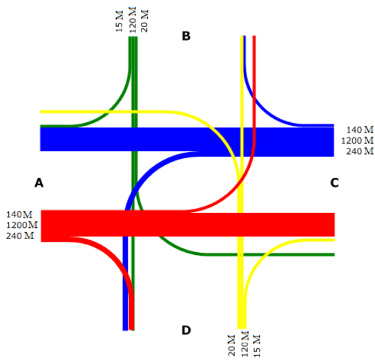
Рисунок 3.22 – Планируемая картограмма интенсивностей движения на перекрестке
