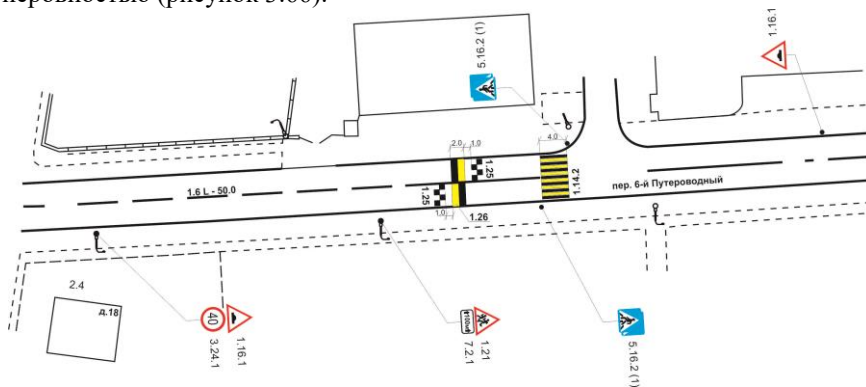
Рисунок 3.66 – План участка улицы с устроенной искусственной неровностью
