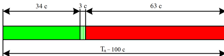
Рисунок 3.69 – Диаграмма работы пешеходного светофора
