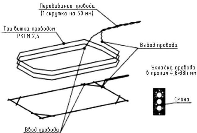
Рисунок 3.85 – Схема выполнения пропилов в асфальтобетонном покрытии
