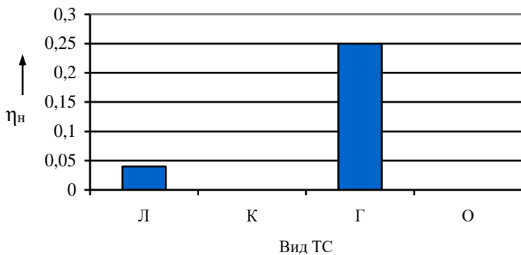
Рисунок 3.80 – Диаграмма коэффициентов нарушений по видам транспортных средств
