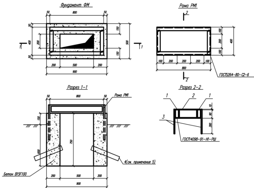
Рисунок 3.47 – Пример чертежа для сооружения фундамента ДК
