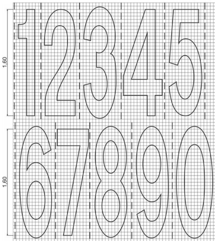
Рисунок В.4 – Цифры для горизонтальной разметки 1.22.1–1.22.3 при скорости движения до 60 км/ч включительно
