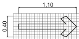
Рисунок В.16 – Горизонтальная разметка 1.33
