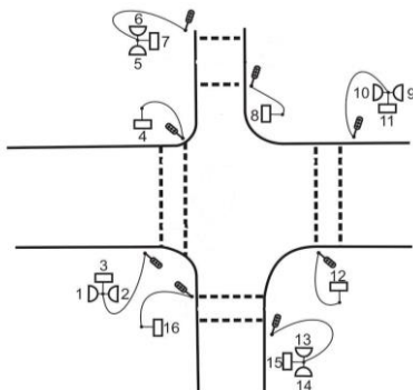
Рисунок 3.36 – Схема нумерации светофоров
