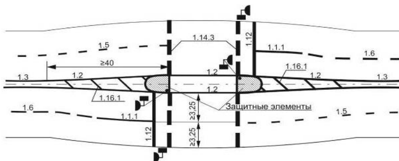
Рисунок 3.10 – Устройство островка безопасности на существующей дороге с изменением ширины полос движения и боковых разделительных полос
