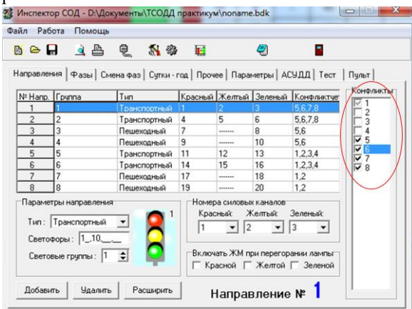
Рисунок 3.41 – Задание недопустимых конфликтов по направлениям
