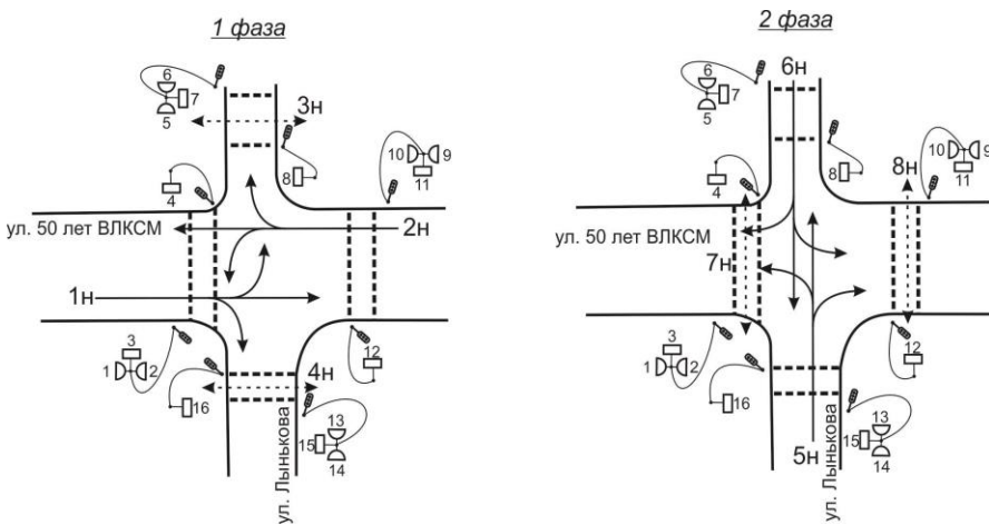
Рисунок 3.37 – Схема пофазного движения на регулируемом перекрестке
