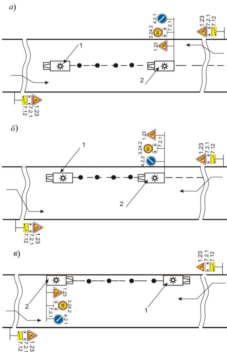
Рисунок 3.62 – Обозначение зоны работ при нанесении линий горизонтальной разметки на проезжей части:
