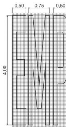
Рисунок В.6 – Буквы для горизонтальной разметки 1.22.1 – 1.22.3 при скорости движения:
