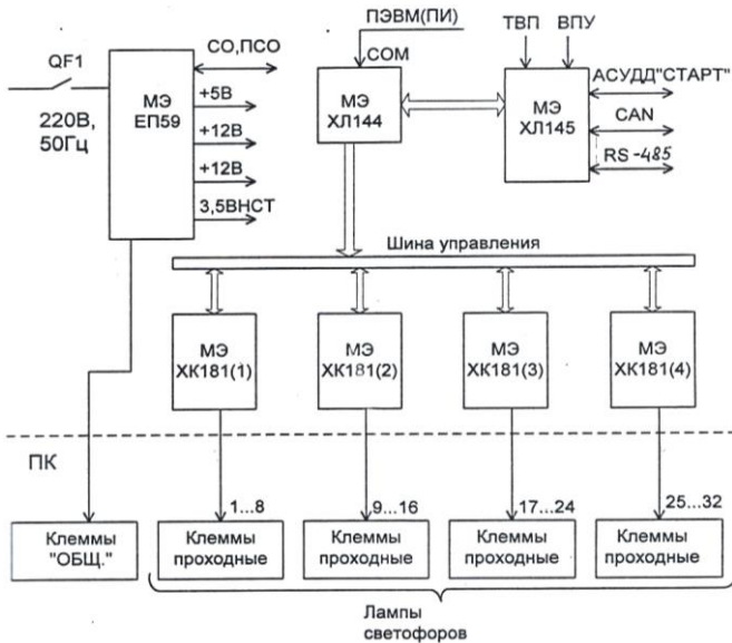
Рисунок 3.34 – Структурная схема БДКЛ-М в вариантах исполнения от БДКЛ-М-8 до БДКЛ-М-32с
