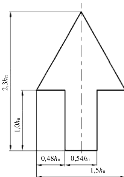
Рисунок 3.13 – Конфигурация стрелок на дорожных знаках 5.20.1, 5.20.2, 5.31 (для поворотных направлений): h_n – высота прописной буквы
