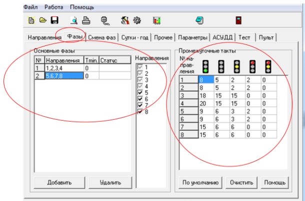
Рисунок 3.42 – Группировка направлений движения по фазам
