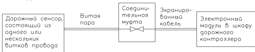
Рисунок 3.82 – Структурная схема детектора индуктивного типа
