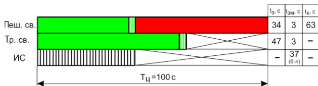
Рисунок 3.77 – Диаграмма работы исследуемых сигналов светофора
