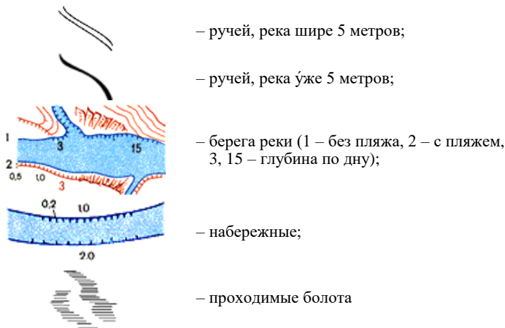
Рисунок 3.3 – Обозначение элементов гидрографии
