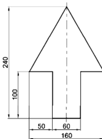
Рисунок 3.16 – Конфигурация стрелок на дорожных знаках 5.29.3
