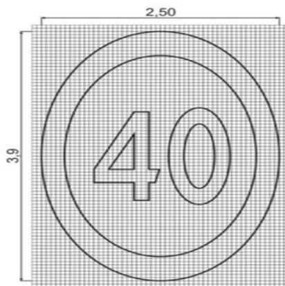
Рисунок В.10 – Горизонтальная разметка 1.27
