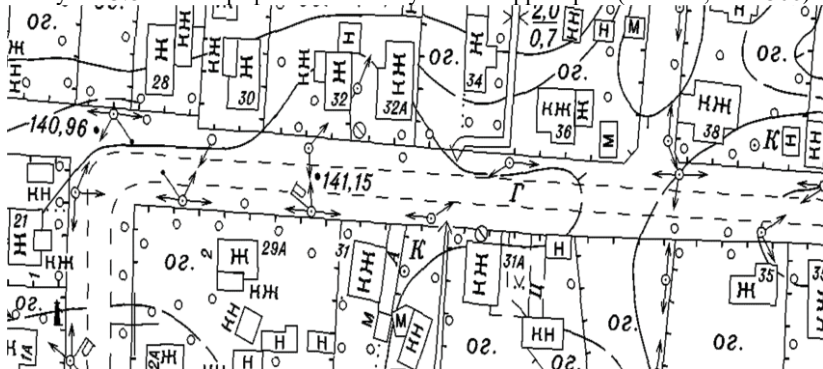
Рисунок 3.9 – Топографический план участка территории (полный, М 1: 2000)
