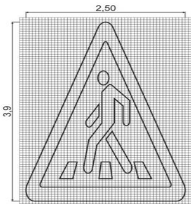
Рисунок В.7 – Горизонтальная разметка 1.24.1
