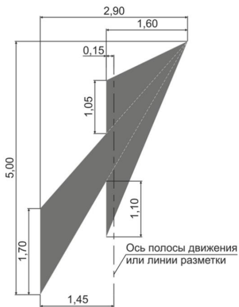
Рисунок В.2 – Горизонтальная разметка 1.19
