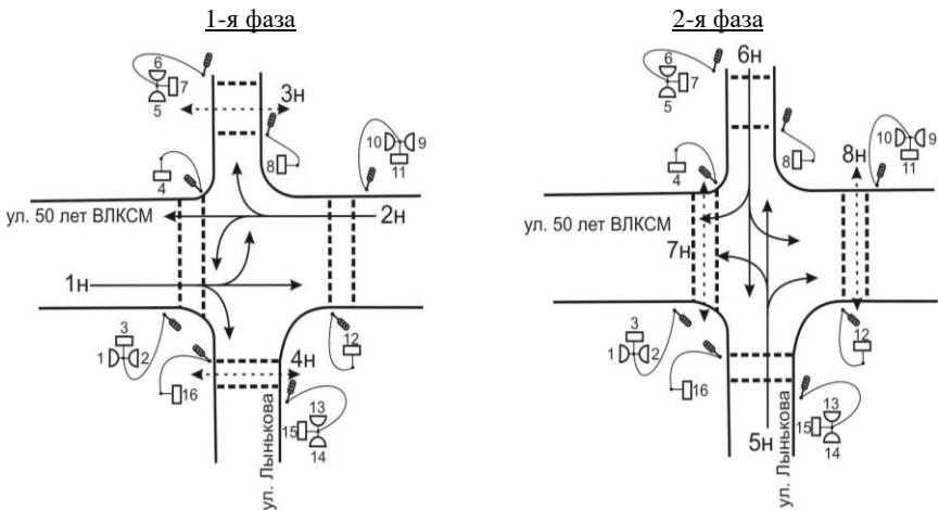
Рисунок 3.26 – Схема пофазного движения
