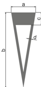
Т а б л и ц а В.3 – Размеры разметки 1.20, обозначенные латинскими буквами
