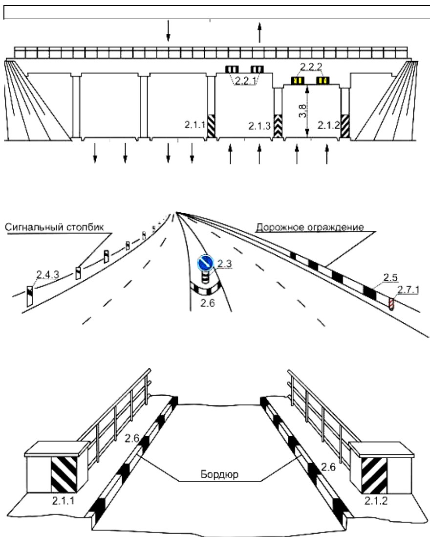
Рисунок В.18 – Примеры применения вертикальной разметки
