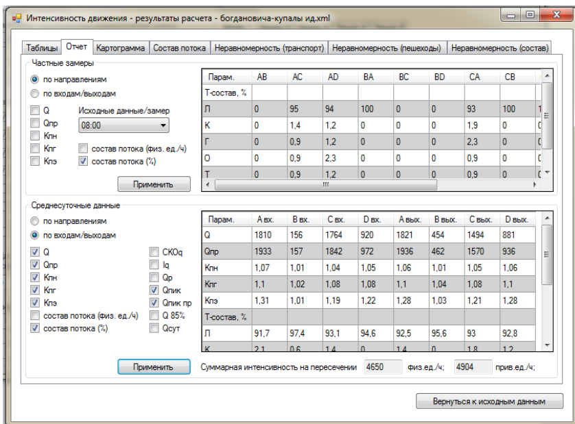
Рисунок 3.54 – Окно «Отчет» с параметрами потоков для отдельных замеров и среднесуточными данными по направлениям и входам/выходам
