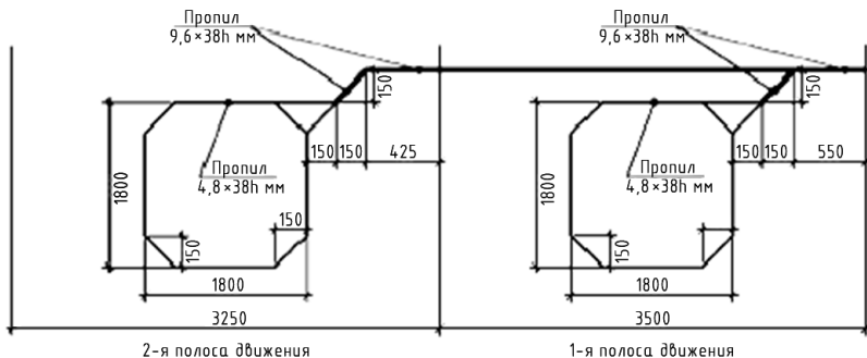
Рисунок 3.84 – Схема выполнения пропилов в асфальтобетонном покрытии
