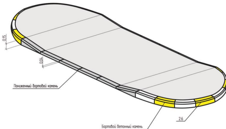
Рисунок 3.11 – Конструкция островка безопасности
