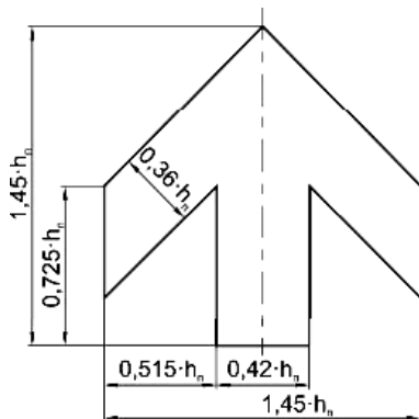
Рисунок 3.15 – Конфигурация стрелок на дорожных знаках 5.21.1, 5.21.2: h_n – высота прописной буквы
