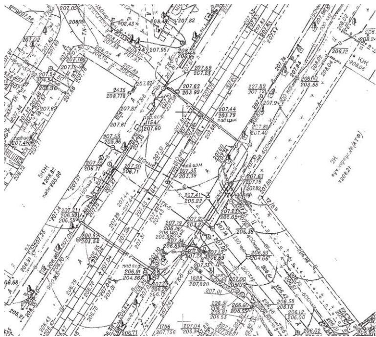
Рисунок 3.8 – Топографический план участка территории (полный, М 1: 500)
