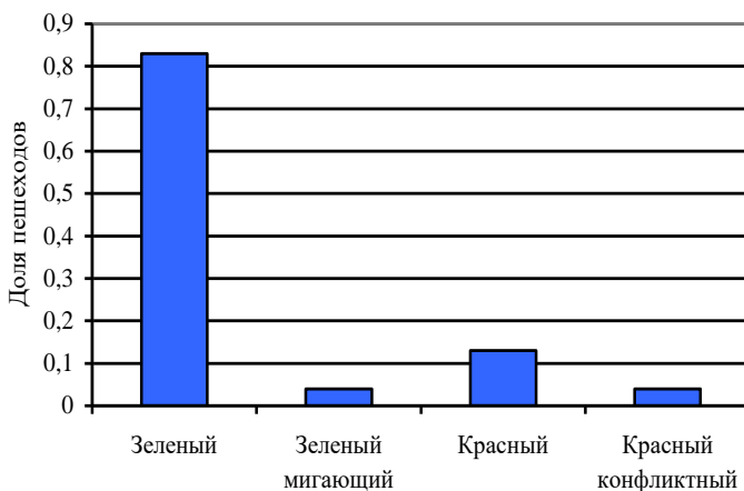
Рисунок 3.71 – Диаграмма распределения пешеходов, завершивших движение при различных сигналах пешеходного светофора
