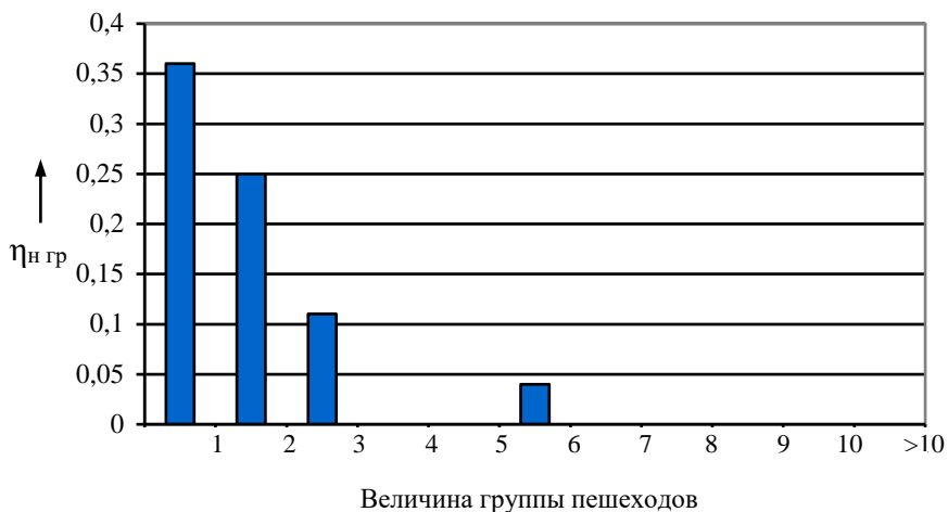
Рисунок 3.81 – Диаграмма коэффициентов нарушений по величине группы пешеходов
