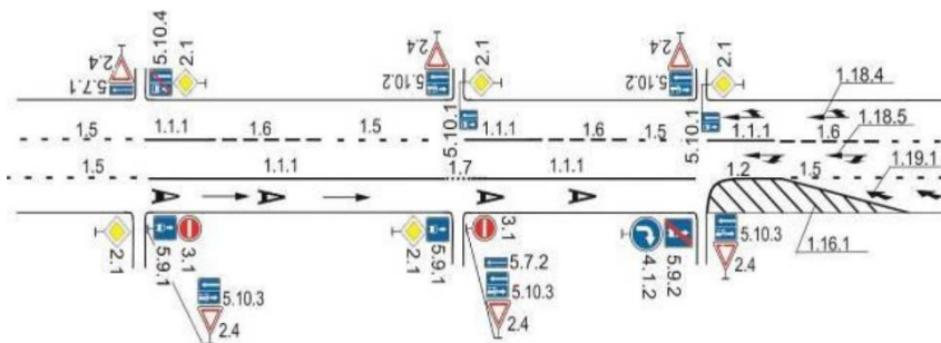
Рисунок 3.23 – Схема применения дорожных знаков и разметки на характерных участках автомобильных дорог, улиц
