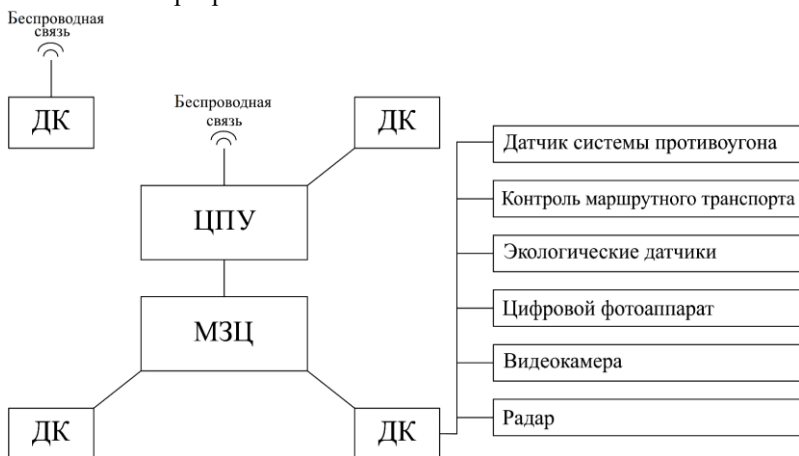
Рисунок 3.33 – Структурная схема АСУДД уровня 4 и выше
