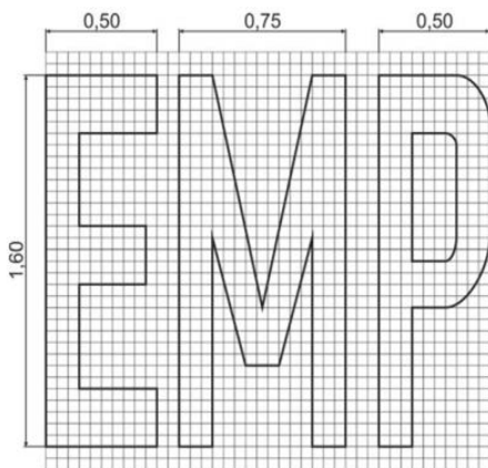
Рисунок В.6 – Буквы для горизонтальной разметки 1.22.1 – 1.22.3 при скорости движения:
