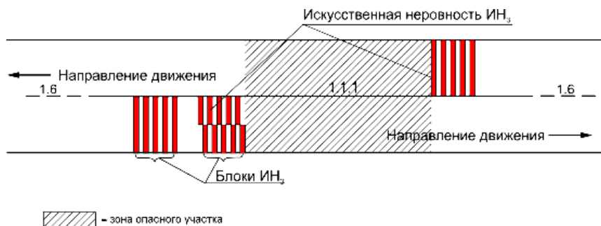
Рисунок 3.65 – Схема размещения блоков ИН 3
