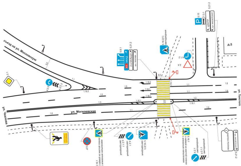
Рисунок 3.12 – План пешеходного перехода с островком безопасности
