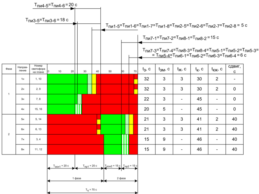
Рисунок 3.28 – Графическое изображение переходных интервалов
