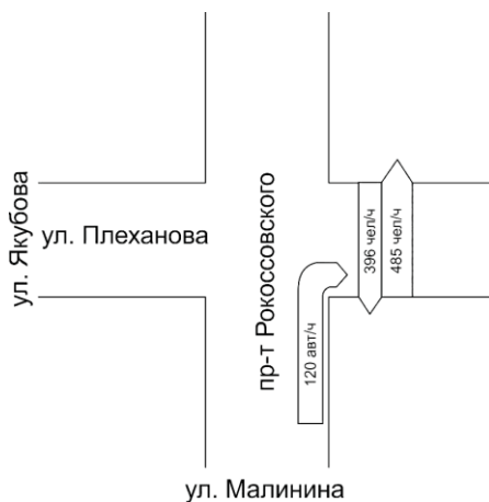
Рисунок 3.78 – Картограмма интенсивностей пешеходного и правоповоротного транспортного потоков
