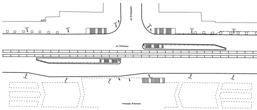
Рисунок 3.6 – Элементы дорожной сети
