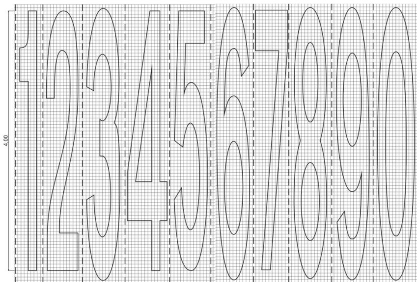
Рисунок В.5 – Цифры для горизонтальной разметки 1.22.1–1.22.3 при скорости движения более 60 км/ч
