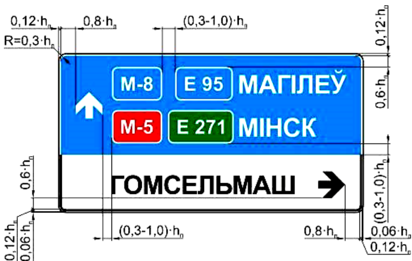
Рисунок А.3 – Пример компоновки изображения знака 5.21.2
