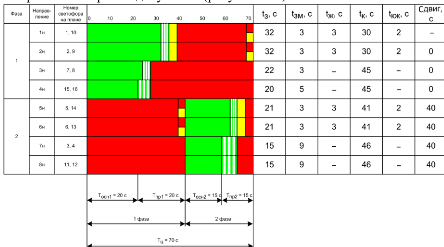
Рисунок 3.39 – Диаграмма светофорного регулирования
