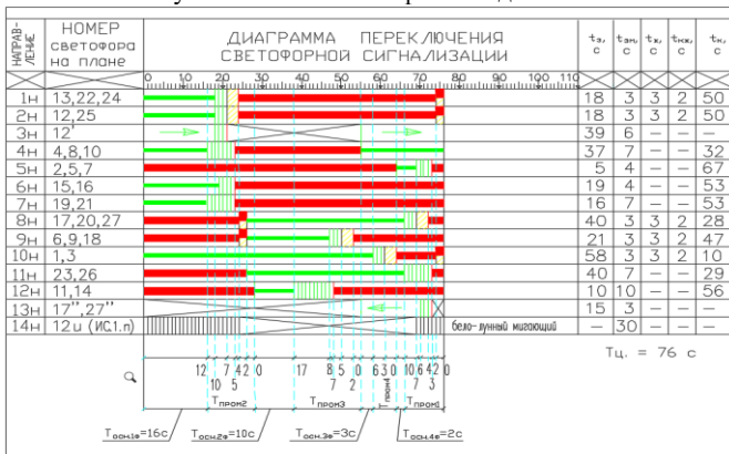
Рисунок 5.1 – Схема пофазного движения
