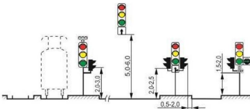
Рисунок 3.25 – Расположение светофоров относительно проезжей части Лабораторная работа № 6
