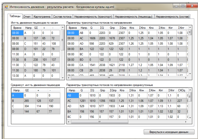
Рисунок 3.53 – Окно «Таблицы параметров транспортных и пешеходных потоков»
