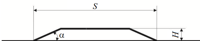
Рисунок 3.64 – Схема конструкции ИН 1 трапециевидной формы
