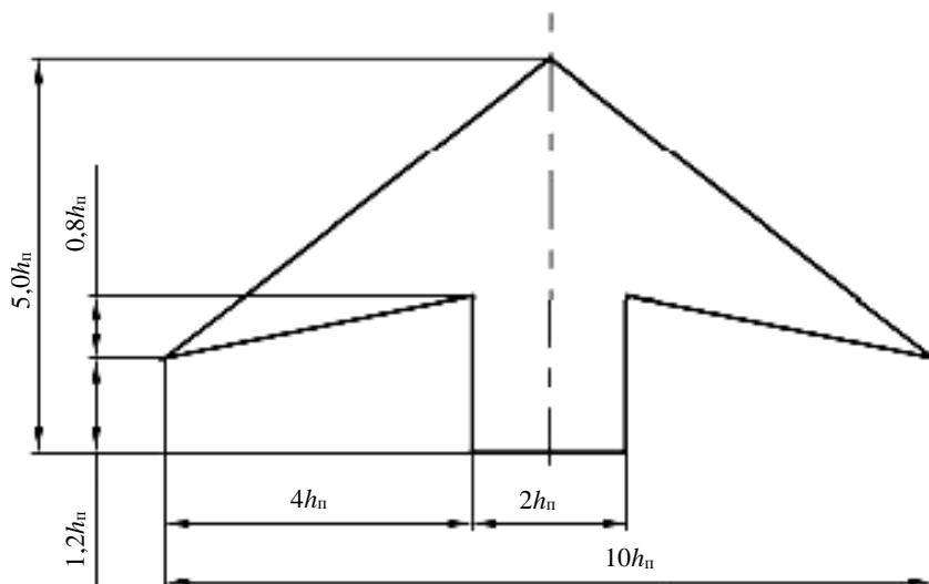
Рисунок 3.14 – Конфигурация стрелок на дорожных знаках 5.20.2 (для прямых направлений): h_n – высота прописной буквы
