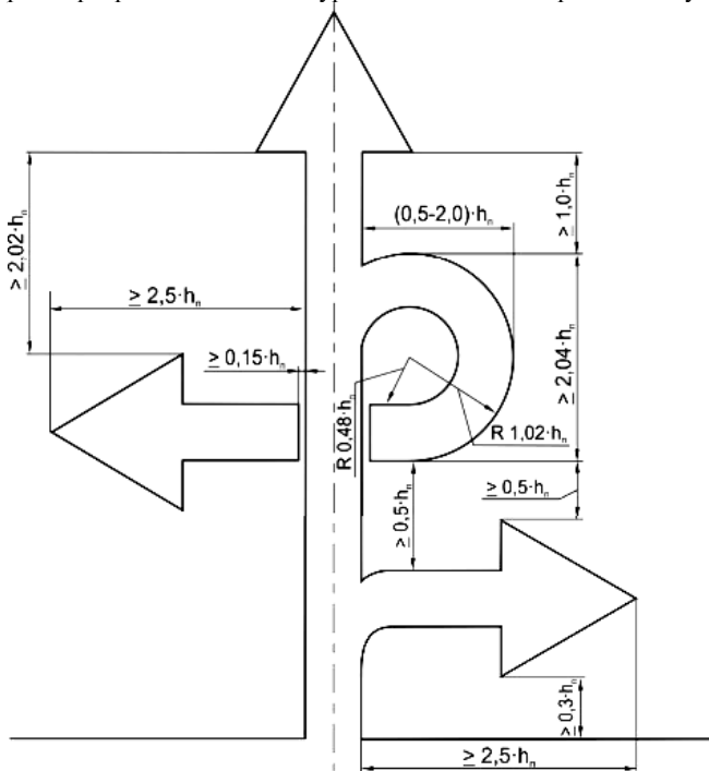
Рисунок 3.17 – Конфигурация стрелок на дорожных знаках 5.20.1, устанавливаемых перед перекрестками в одном уровне: h_n – высота прописной буквы
