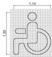
Рисунок В.10 – Горизонтальная разметка 1.27
