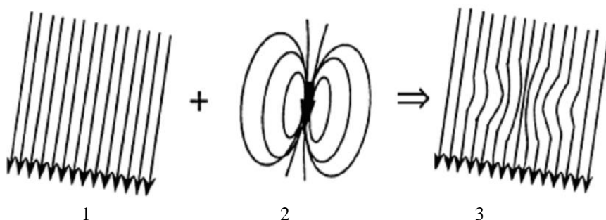
Рисунок 4.2 – Влияние стороннего магнитного поля на магнитное поле Земли: 1 – магнитное поле Земли при отсутствии магнитных предметов; 2 – магнитный диполь, создаваемый магнитными материалами; 3 – результирующее магнитное поле
