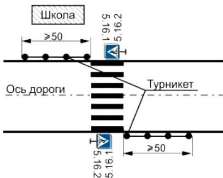
Рисунок 3.24 – Пример установки турникета в местах расположения учебных заведений и предприятий
