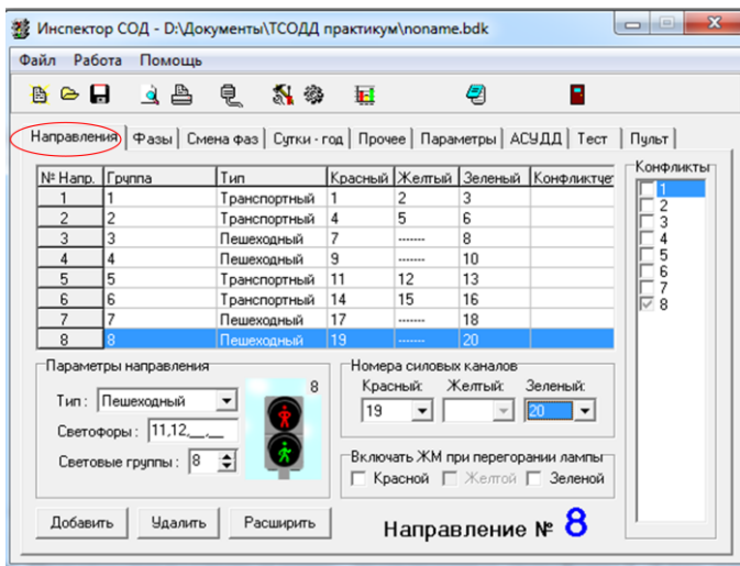
Рисунок 3.40 – Задание направлений движения
