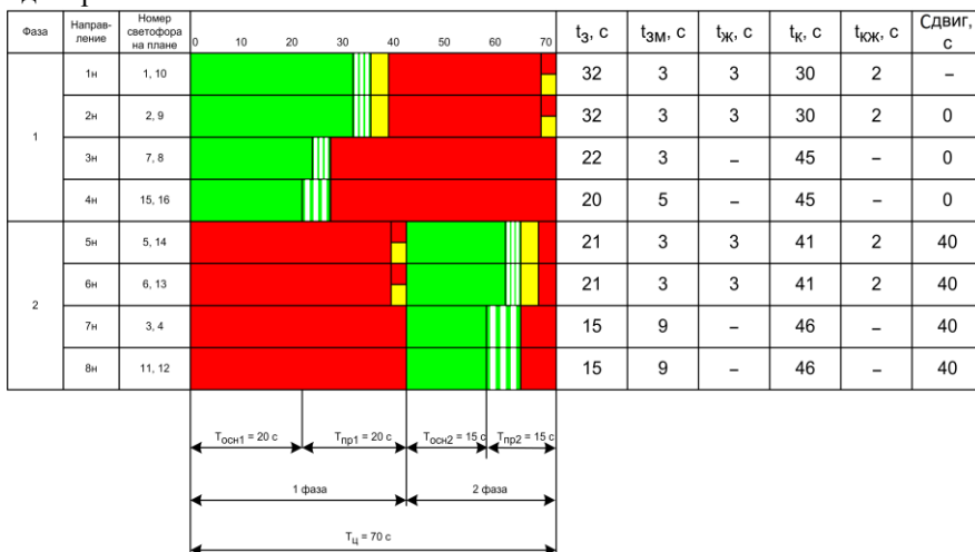
Рисунок 3.27 – Пример диаграммы светофорного регулирования
