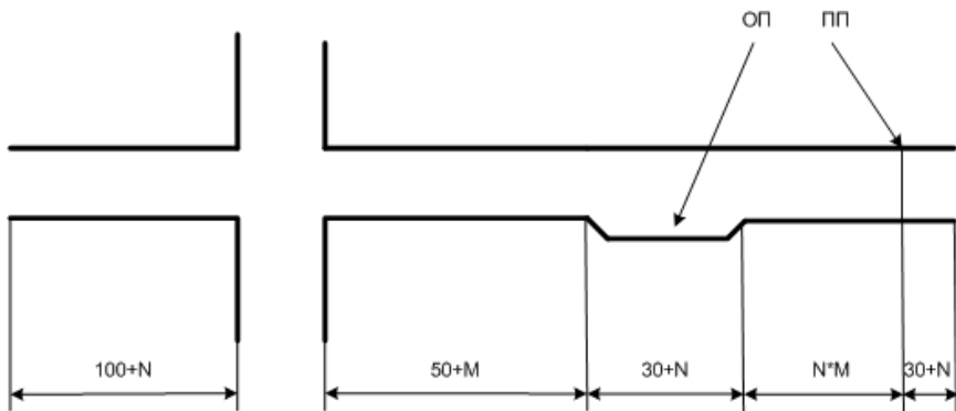
Рисунок 3.21 – Схема участка городской улицы:
