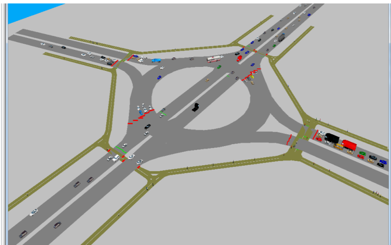
Рисунок 4.8 (окончание) – Визуализация движения конфликтующих потоков на пл. Бангалор в г. Минске:
