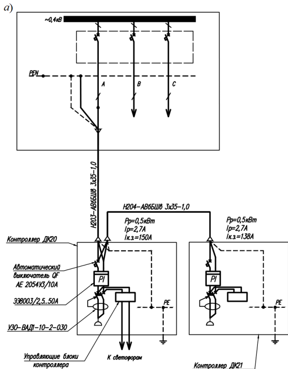
Рисунок 3.50 – Пример схемы электроснабжения ДК и кабельного журнала: а – схема электроснабжения; б – кабельный журнал
