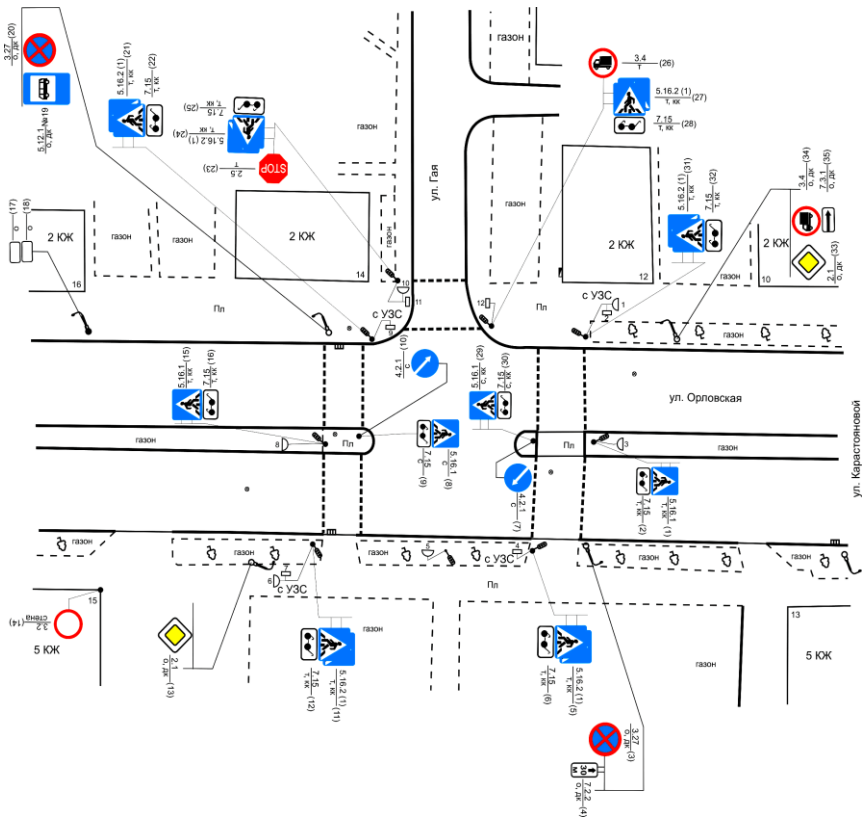
Рисунок 3.20 – План участка улицы с дислокацией пешеходных переходов, ДЗ и СФО
