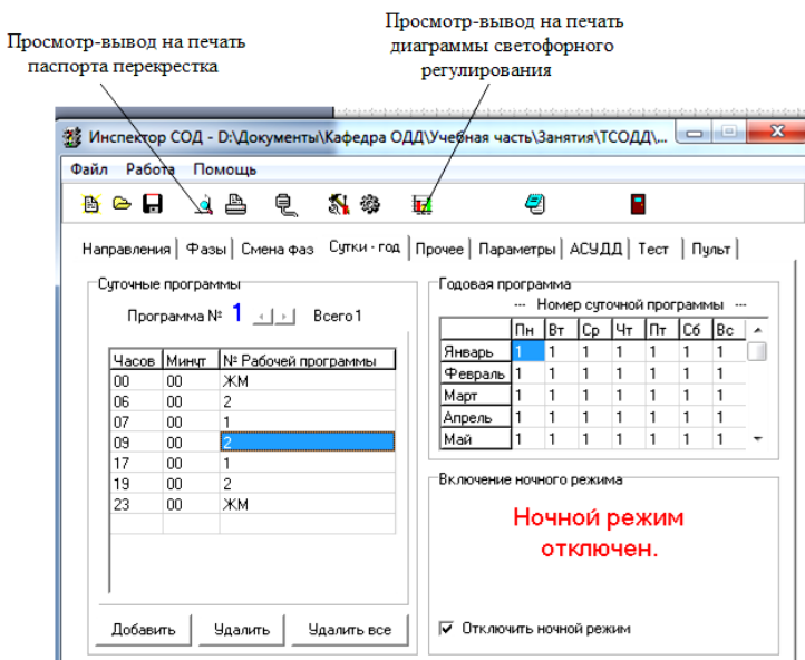
Рисунок 3.46 – Вывод на печать результатов
