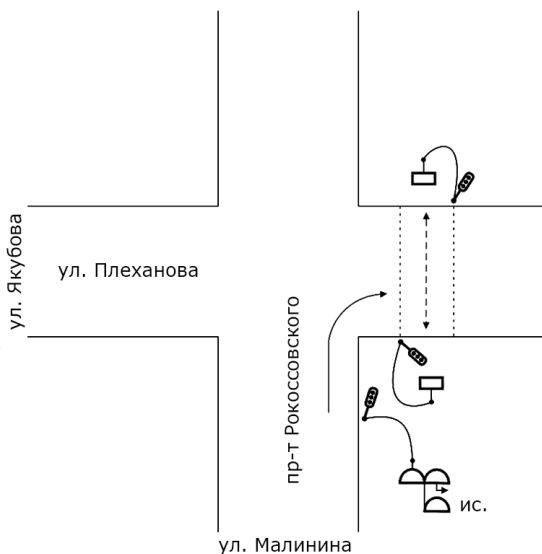
Рисунок 3.76 – Схема исследуемого участка дорожной сети
