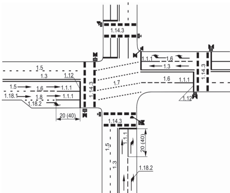
Рисунок 3.61 – Примеры нанесения горизонтальной разметки
