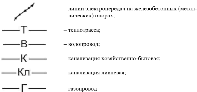
Рисунок 3.5 – Обозначение подземных коммуникаций
