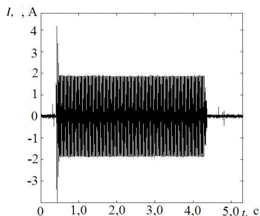
Рисунок 2 – Ток в рабочей цепи стрелочного электропривода переменного тока при переводе исправной одиночной стрелки
