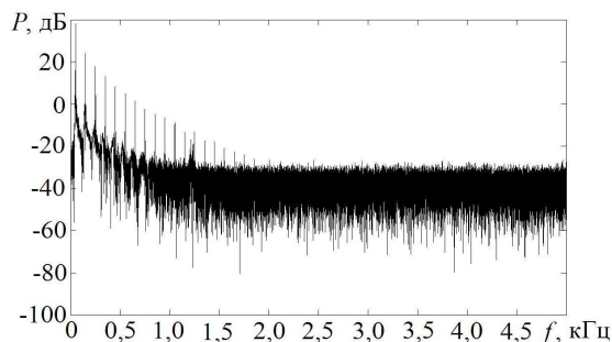
Рисунок 3 – Спектр амплитуды тока в рабочей цепи стрелочного электропривода переменного тока при переводе исправной одиночной стрелки
