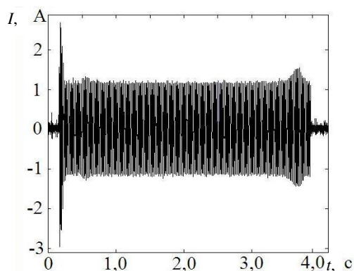
Рисунок 4 – Ток в рабочей цепи стрелочного электропривода переменного тока при переводе одиночной стрелки с упором корня острияка
