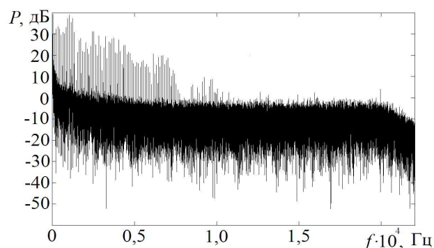
Рисунок 5 – Спектр амплитуды тока в рабочей цепи стрелочного электропривода переменного тока при переводе одиночной стрелки с неисправным ротором
