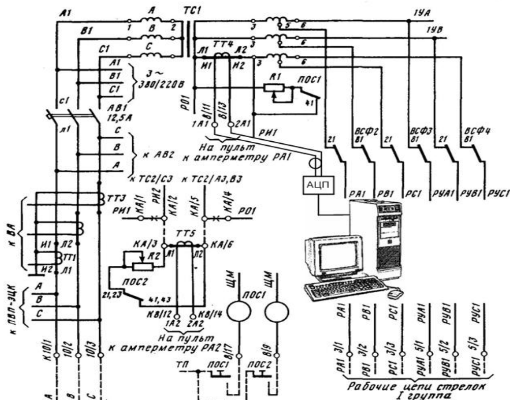
Рисунок 1 – Подключение измерительного устройства к схеме стрелочной панели ПСТ-ЭЦК
