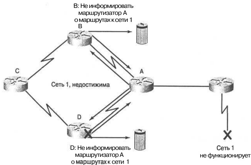
Рис. 12.19. В ситуации, когда используется расщепление горизонта, маршрутизатор, который получил маршрутную информацию через некоторый интерфейс, не посылает вновь информацию об этом маршруте на этот интерфейс
