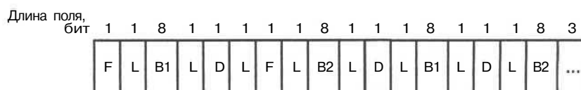
NT-фрейм (от сети к терминалу)
