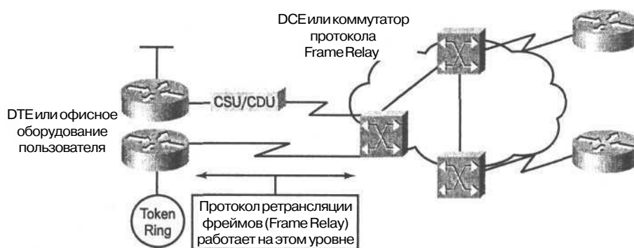
Рис. 12.1. Протокол ретрансляции фреймов (Frame Relay) определяет процесс установки соединения между маршрутизатором и коммутирующим оборудованием локального доступа, используемым провайдером услуг
