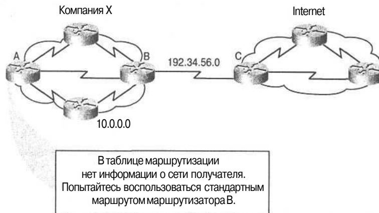
Рис. 1.16. Стандартные маршруты могут быть установлены заданной сетевым администратором статической конфигурацией. Вместо поддержания конкретной информации о топологии сети каждый маршрутизатор компании X проинформирован о маршруте по умолчанию и может получить доступ к любому неизвестному пункту назначения, направив пакет в Internet
