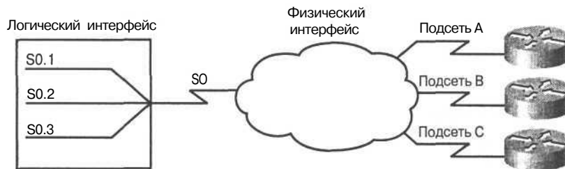
Рис. 12.16. Сообщения об изменениях маршрутной информации могут рассылаться через подынтерфейсы так, как если бы они исходили от различных физических интерфейсов
