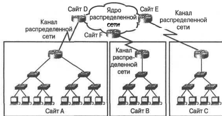
Рис. 9.6. В двухуровневых проектах для создания отдельных логических сетей могут организовываться виртуальные локальные сети
