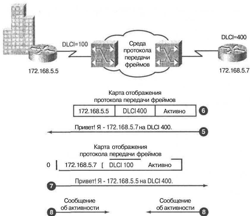
Рис. 12.15. Маршрутизатор изменяет статус каждого DLCI, основываясь на ответе коммутатора протокола ретрансляции фреймов
