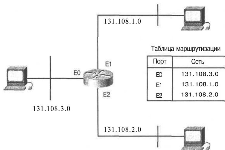
Рис. 4.23. Маршрутизатор структурирует сеть, разделяя сети на подсети
