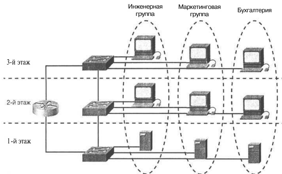
Рис. 4.22. Виртуальные локальные сети сдерживают широковещание и повышают безопасность
