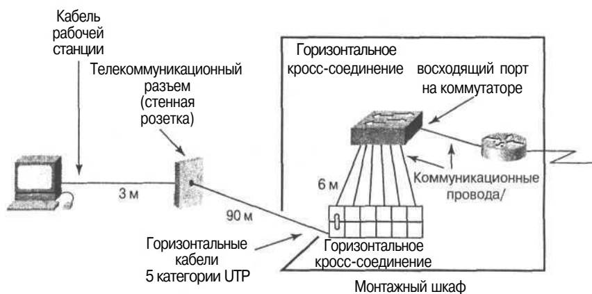
Рис. 4.7. Количество горизонтальных кабельных трасс и размер (количество портов) горизонтальных коммутационных панелей должны быть определены в соответствии с требованиями пользователей
