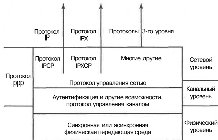
Рис. 10.3. Протокол PPP представляет собой протокол канального уровня со службами сетевого уровня
