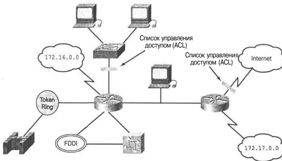
Рис. 6.1. Использование списков управления доступом позволяет выполнить тестирование пакетов на основе адресации или типа потока данных и на этой основе разрешить или запретить доступ потока данных на маршрутизатор или выход с него
