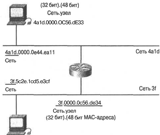
Рис. 7.3. Каждое устройство в сети IPX имеет свой уникальный адрес
