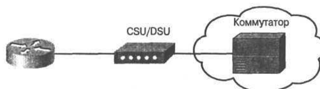
Рис. 8.8. В распределенной сети CSU/DSU размещаются между коммутатором и терминалом
