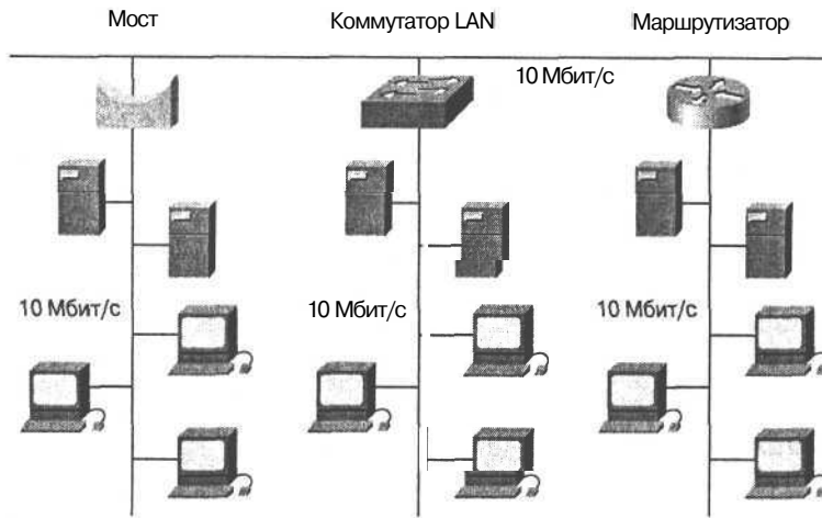
Рис. 2.4. В неsegmentированной сети всем 15 устройствам пришлось бы использовать одну и ту же полосу пропускания в 10 Мбит/с и находиться в одном и том же коллизийном домене
