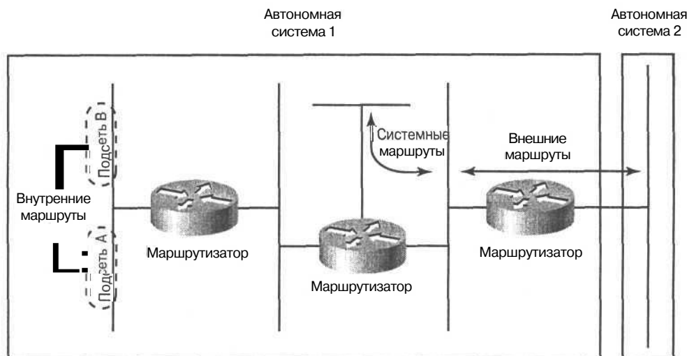
Рис. 5.3. Автономные системы разделены границами областей
