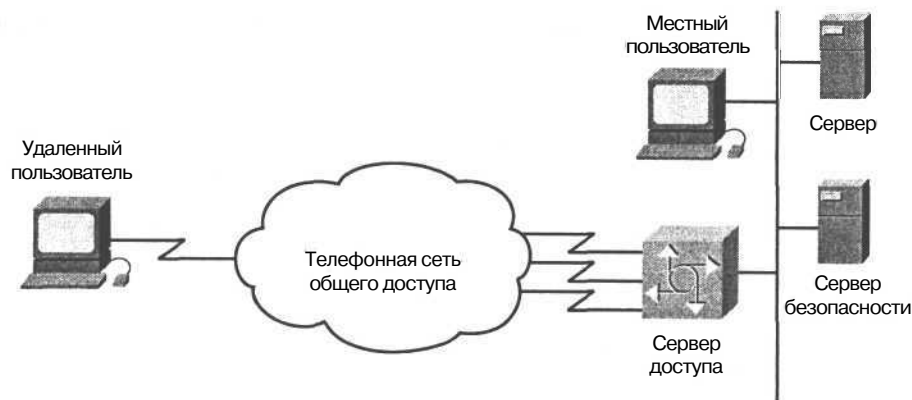
Рис. 11.8. При использовании ISDN удаленный пользователь может считаться обычным локальным сетевым узлом
