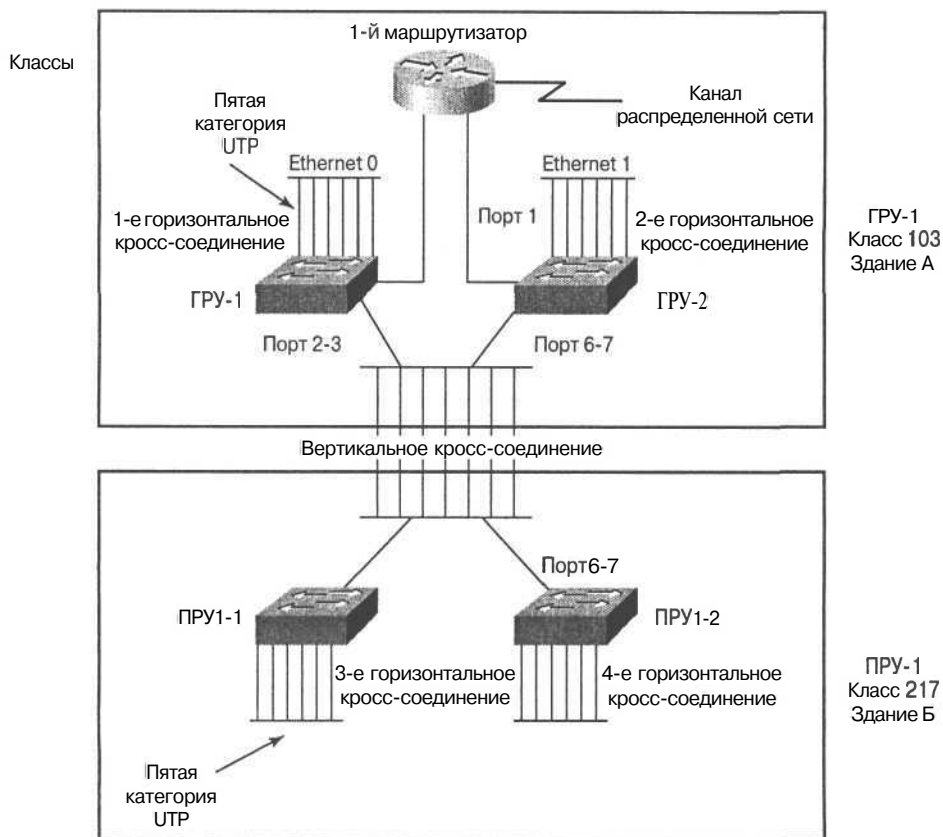
Рис. 4.27. Физическая карта показывает, где находятся ГРУ и ПРУ, а также точки подключения хостов к сети
