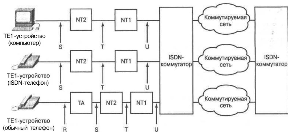
Рис. 11.3. Несколько устройств могут получить доступ к различным типам сетей через ISDN-коммутатор
