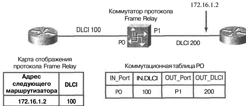
Рис. 12.11. Маршрутизатор узнает используемые DLCI от коммутатора протокола ретрансляции фреймов и посылает запрос инверсного ARP каждому DLCI
