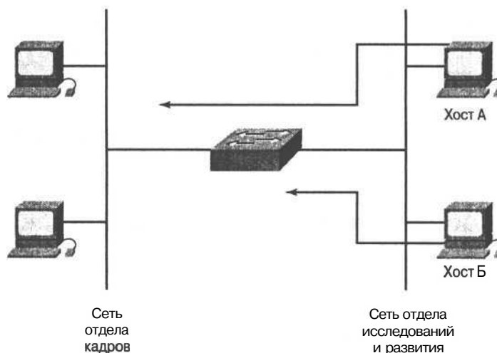
Рис. 6.2. Использование списков управления доступом позволяет предотвратить направление потока данных в какую-либо сеть
