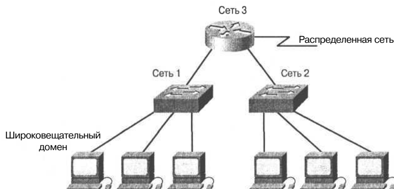
Рис. 4.20. Маршрутизация 3-го уровня решает такие вопросы, как необходимость физического разделения подсетей
