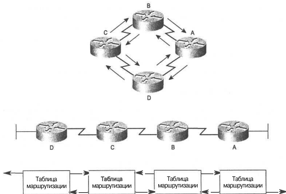
Рис. 1.17. Регулярный обмен информацией между маршрутизаторами отображает изменения в топологии сети
