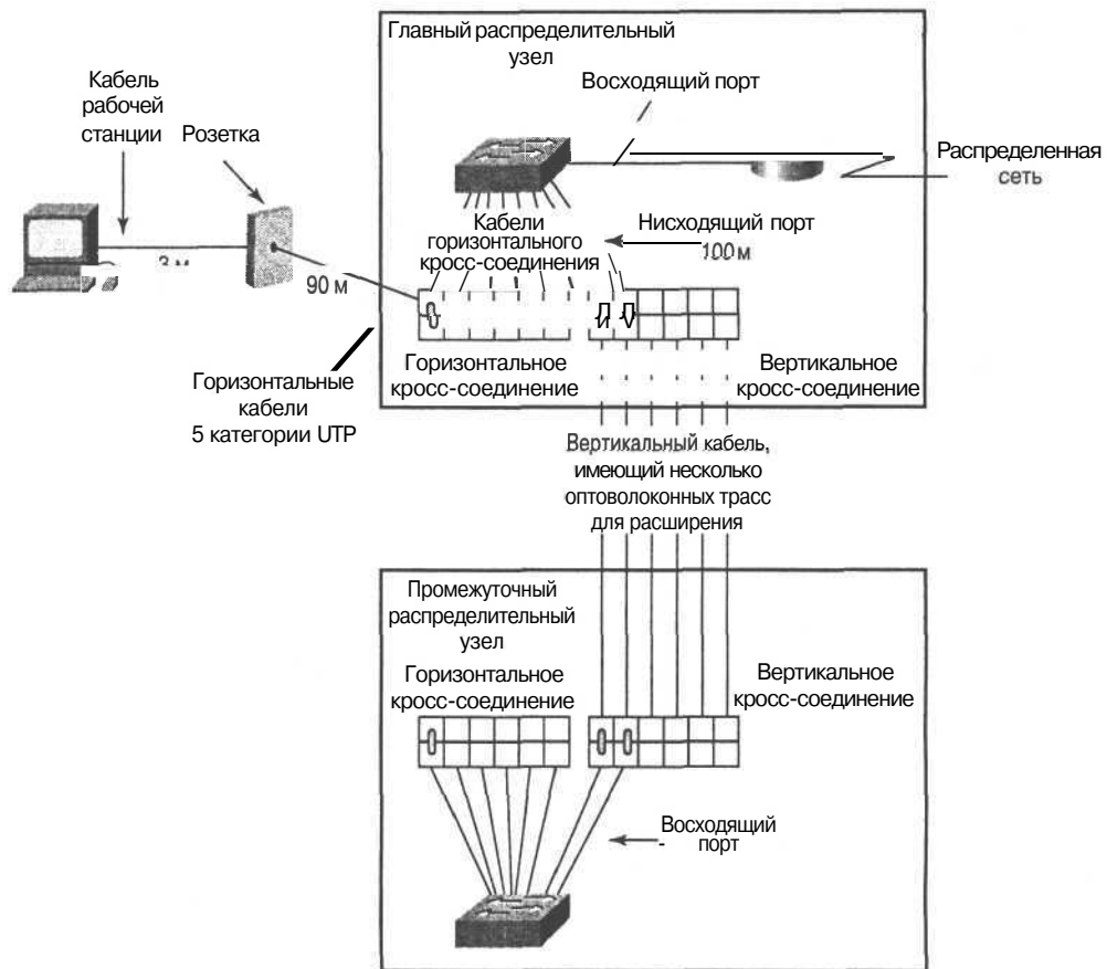
Рис. 4.9. Основное отличие между ГРУ и ПРУ — это появление дополнительной коммутационной панели, которая может быть вертикальным кросс-соединением
