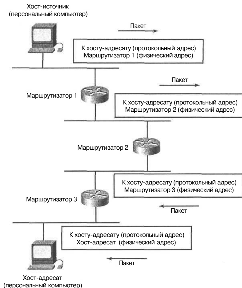
Рис. 5.1. При движении пакета по сети его физический адрес меняется, но протокольный адрес остается неизменным
