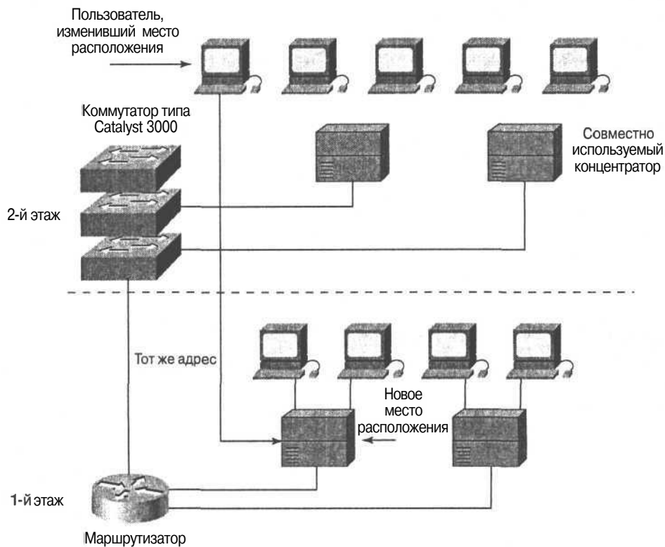
Рис. 3.6. Коммутаторы, способные создавать виртуальные сети, значительно упрощают решение проблем, связанных с изменением схемы прокладки кабелей, конфигурации сети, с переездом пользователя в другое место, а также задач отладки при повторном подключении пользователя к сети
