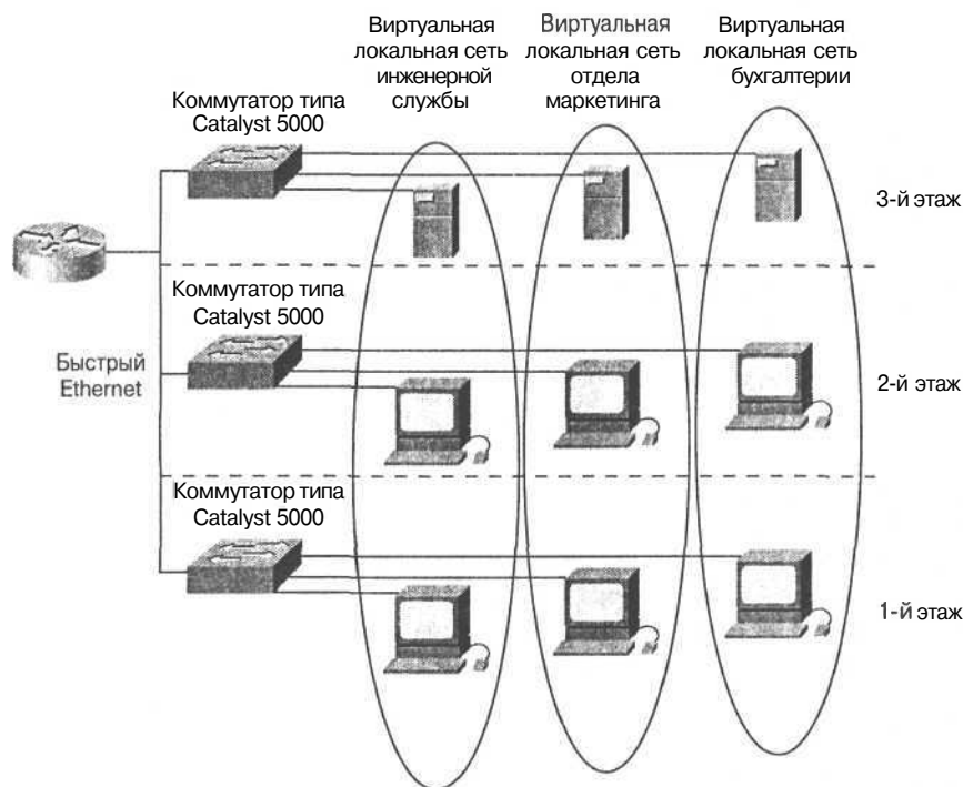
Рис. 3.3. Использование виртуальных сетей позволяет ликвидировать ограничения на обмен информацией между рабочими группами
