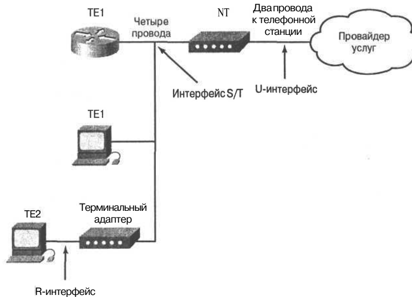
Рис. 8.18. ISDN представляет собой цифровую сетевую технологию, используемую для передачи голосовых, цифровых, факс-модемных и видеоданных от одного конца сети к другому
