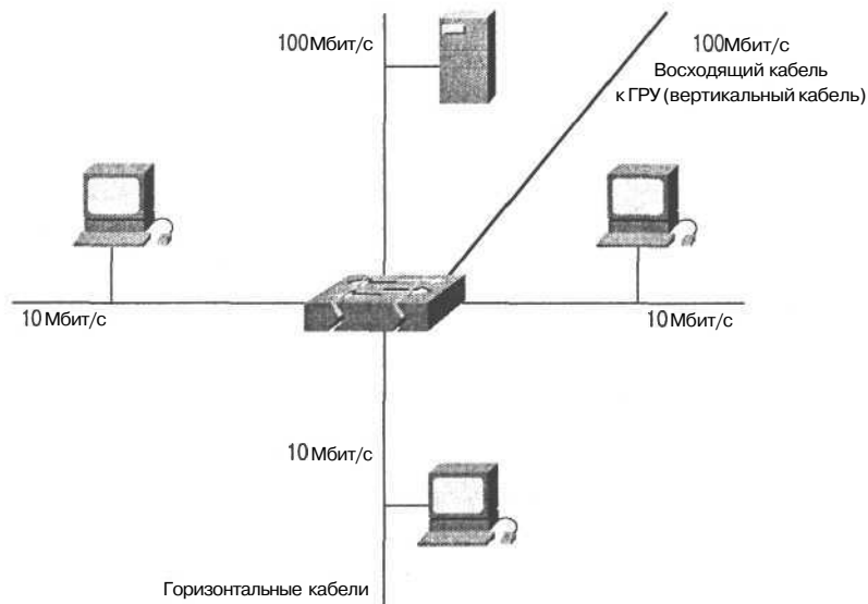
Рис. 4.14. Пример асимметричной коммутации
