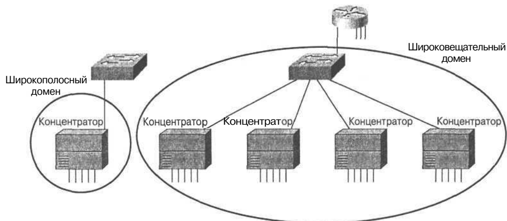
Рис. 4.4. Коллизийный домен имеет общую полосу пропускания и называется широкополосным, а широковещательный домен виден всей подсети
