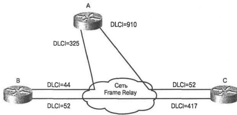
Рис. 12.6. Два конечных устройства на разных концах соединения могут использовать различные номера DLCI для обращения к одному и тому же соединению
