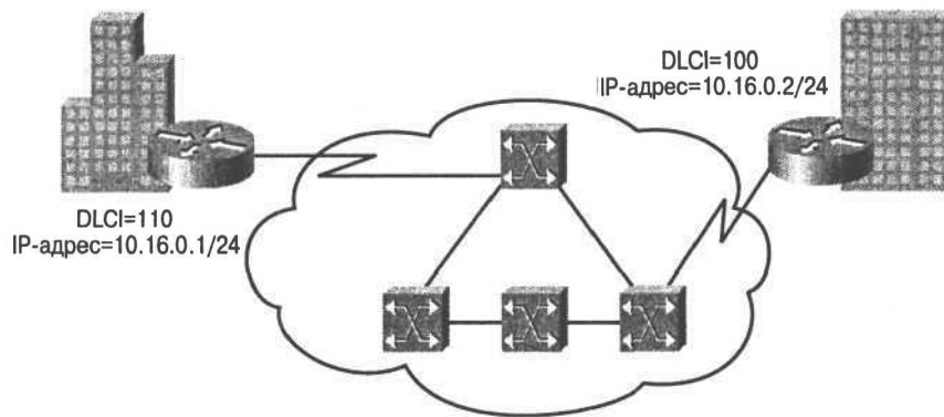
Рис. 12.25. Ответы на запросы инверсного ARP об адресе следующего перехода заносятся в таблицу отображения инверсного протокола ARP
