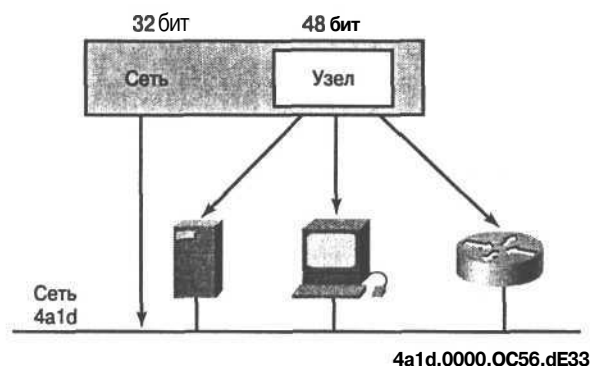
Рис. 7.2. Формат 80-битового адреса протокола Novell IPX; из них 32 бита отводится под номер сети и 48 битов — под номера узла
