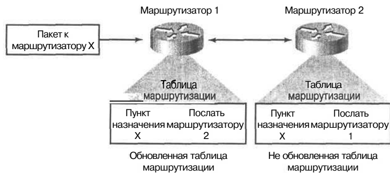
Рис. 5.2. Петля в процессе маршрутизации существует до тех пор, пока не будет обновлена информация о сети или не будет достигнут допустимый максимум коммутаций
