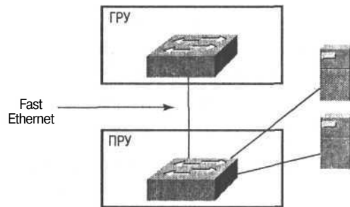
Рис. 4.11. Fast Ethernet соединяет ГРУ и ПРУ, используя 100 Мбит/с полосу пропускания и технологию CSMA/CD
