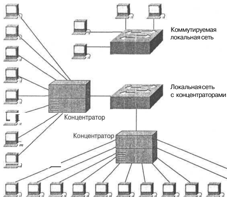
Рис. 4.17. В идеальной локальной сети размер коллизийного домена равен 2. В сети, использующей концентраторы, коллизийный домен становится значительно больше
