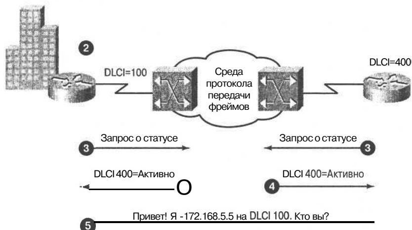
Рис. 12.14. Если инверсный ARP не работает или удаленный маршрутизатор не поддерживает этот протокол, то необходимо сконфигурировать маршруты (т.е. DLCI и IP-адреса) удаленных маршрутизаторов
