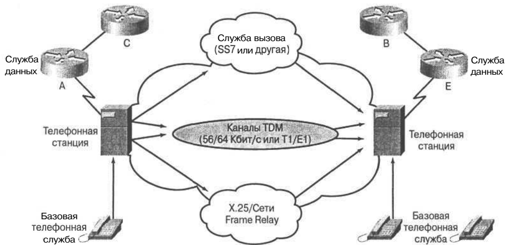
Рис. 8.2. В распределенных сетях имеется три типа провайдеров услуг
