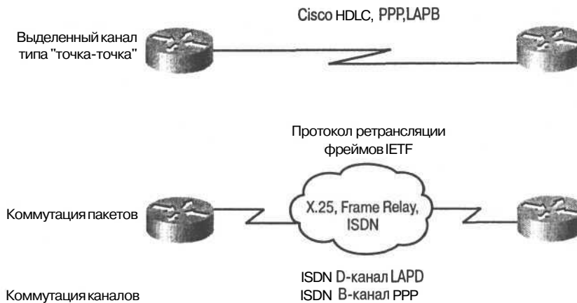
Рис. 8.11. Выбор протокола инкапсуляции зависит от технологии распределенной сети и от типа оборудования, осуществляющего связь
