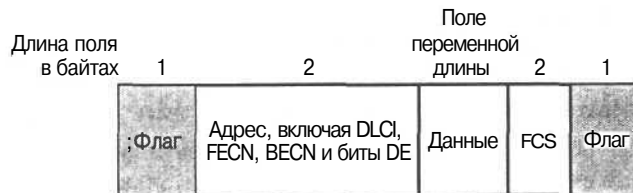
Рис. 12.7. Поля флагов задают начало и конец фрейма
