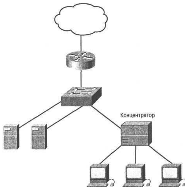
Рис. 4.15. Используя микросегментацию для устранения коллизионных доменов, можно избежать перегрузок в локальной сети
