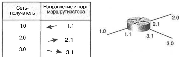
Рис. 1.15. Маршрутизатор передает пакет в следующую сеть по заданному пути, а сетевую часть адреса использует для выбора пути
