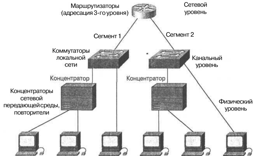
Рис. 4.3. Для сегментации сети используются маршрутизаторы и коммутаторы
