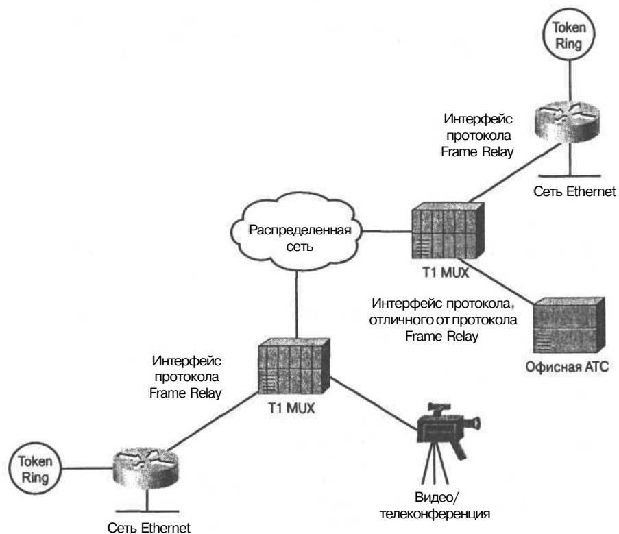
Рис. 12.4. Протокол Frame Relay может использоваться в качестве интерфейса к сети за счет соединения между собой таких устройств, как коммутаторы этого протокола и маршрутизаторы
