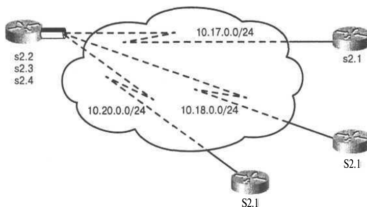
Рис. 12.24. В конфигурации подынтерфейса типа point-to-point подынтерфейс функционирует как выделенная линия
