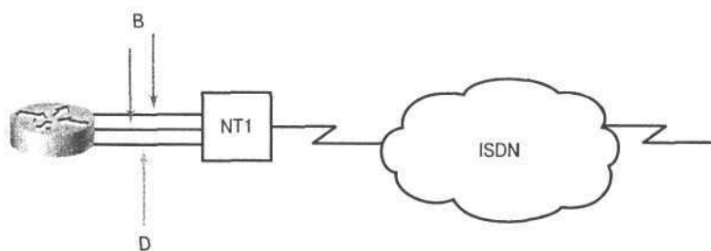
Рис. 11.12. BRI, используемый для служб ISDN, предлагает два В-канал и один D-канал
