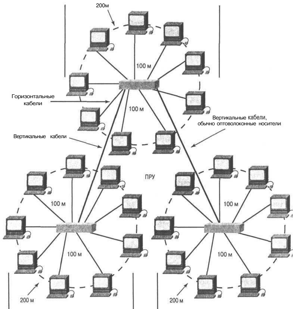
Рис. 4.10. Все вертикальные кабели подсоединяются к ГРУ для создания одного сегмента локальной сети
