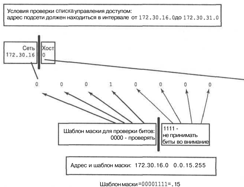
Рис. 6.7. Адрес 172.30.16.0 с шаблоном маски 0.0.15.255 соответствует сетям с номерами от 172.30.16.0 до 172.30.31.0
